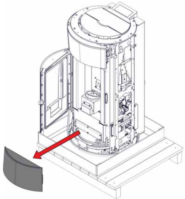
Frontplatte demontiert
