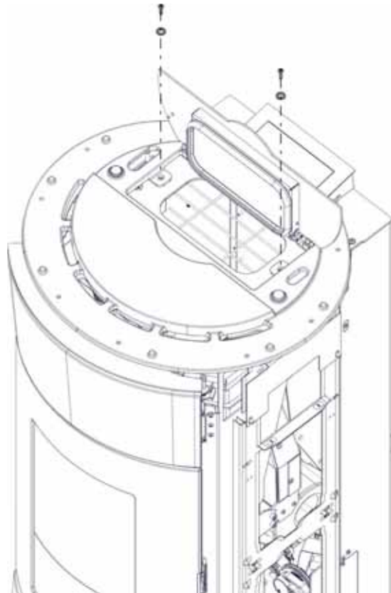
1) Pellettank öffnen und Schrauben abschrauben
