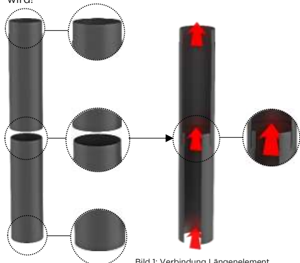
Bild 1: Verbindung Längenelement
