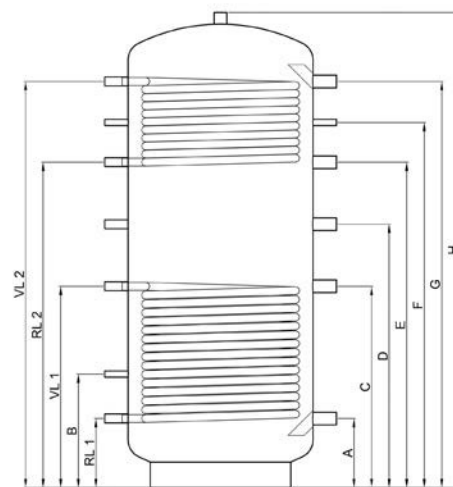
Pufferspeicher Typ PR-2 (mit zwei Wärmetauschern)
