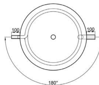
Pufferspeicher Typ PR-2 (mit zwei Wärmetauschern)
