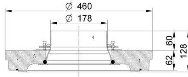
Speicherringe für Abgang oben
