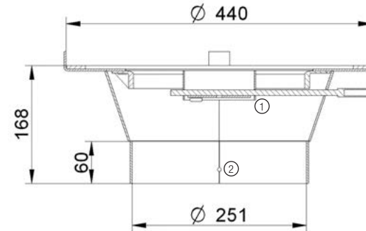
Konzentrischer Adapter „K“
