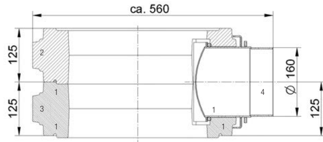
Speicherringe für seitlichen Abgang
