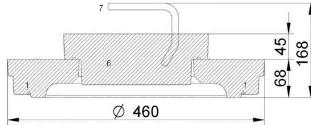
Stopfen und Henkel
