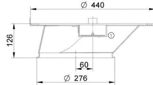
Gerader Adapter „G“
