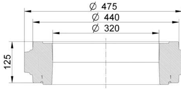
Speicherring geschlossen
