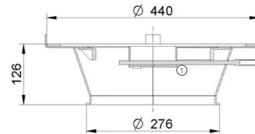
Konzentrischer Adapter „K“
