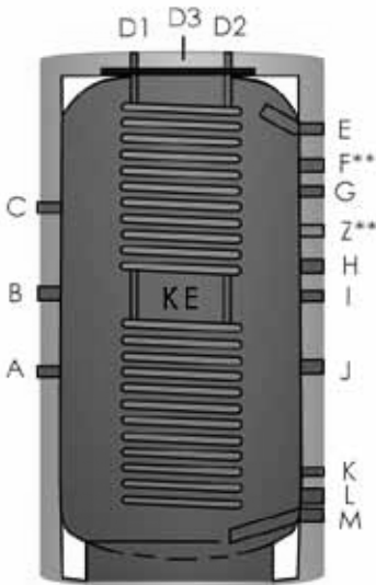
Hygienespeicher ohne Wärmetauscher
