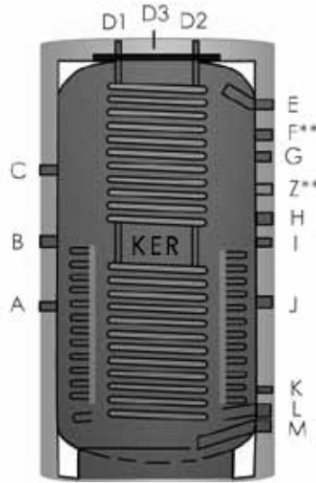
Hygienespeicher mit einem Wärmetauscher
