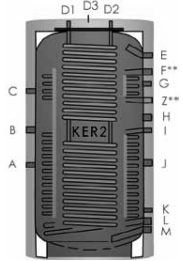
Hygienespeicher mit zwei Wärmetauschern
