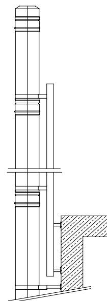
Bild 12: Aufbau mit Kragarm
