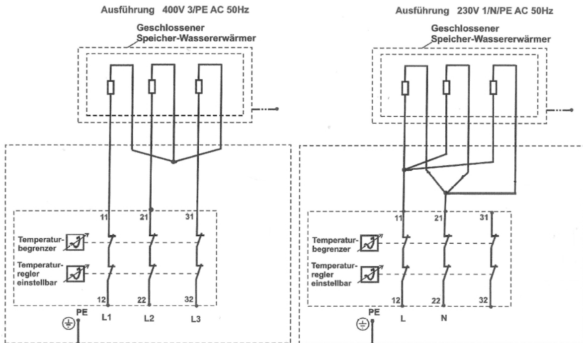
Schaltbild Einschraubheizkörper
