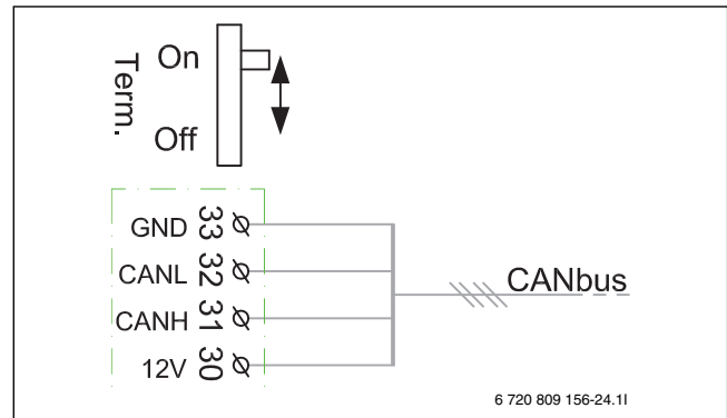
Bild 8 CAN-BUS-Terminierung
