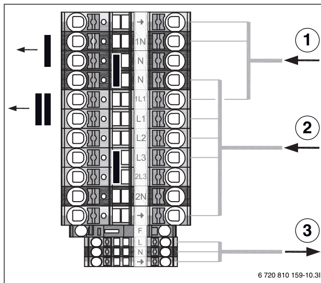
Bild 33 Klemmenanschlüsse und Anordnung der Brücken
