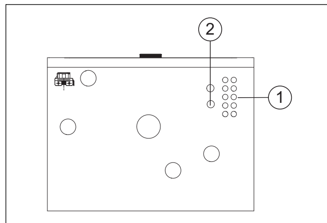
Bild 10 Kabeldurchführungen
