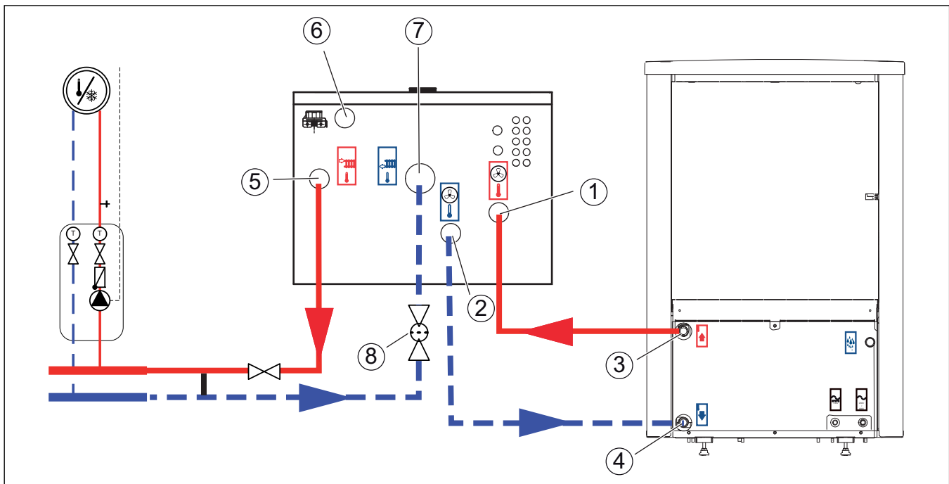
Bild 6 Anschluss des Inneneinheits mit elektrischem Zuheizung an Wärmepumpe und Heizungsanlage
