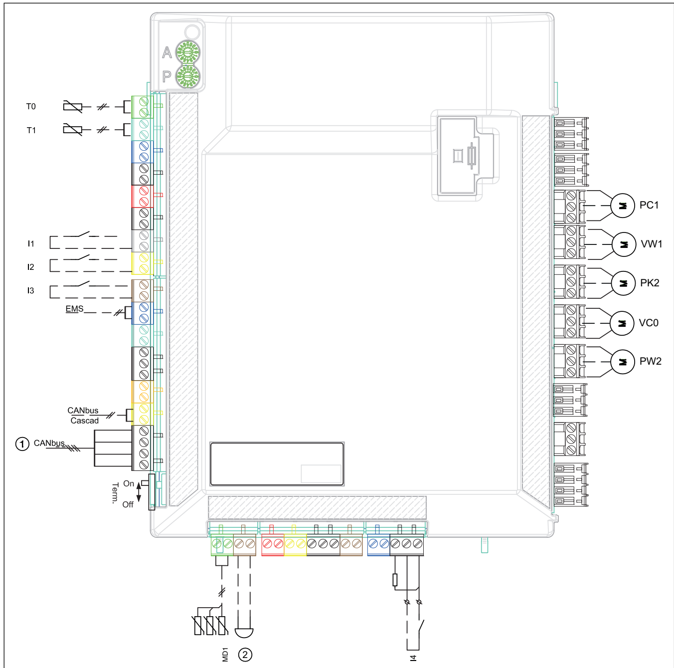
Bild 12 Anschlüsse Installationsmodul
