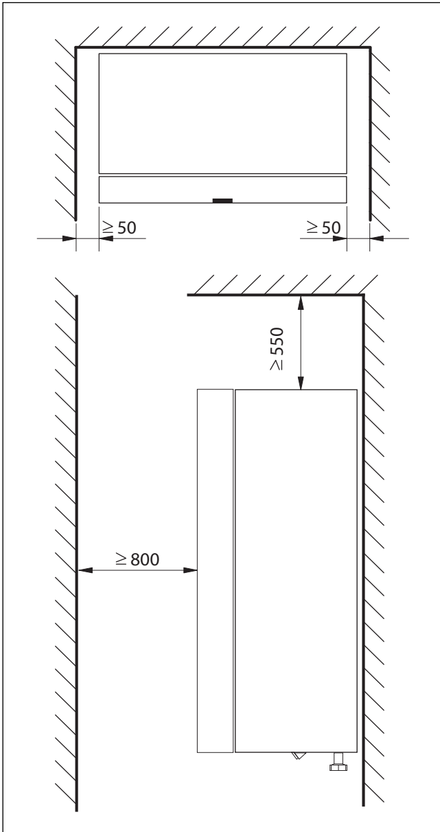
Bild 3 Mindestabstand (mm)
