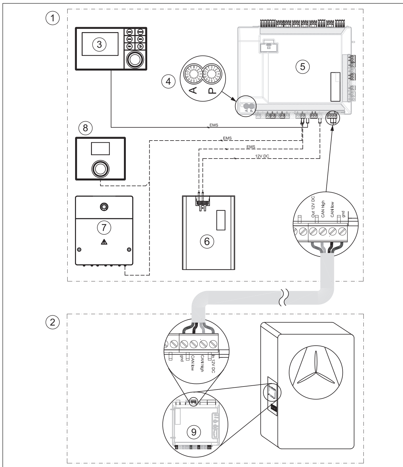
Bild 28 CAN-BUS/EMS-BUS für Inneneinheit mit elektrischem Zuheizter – Überblick
