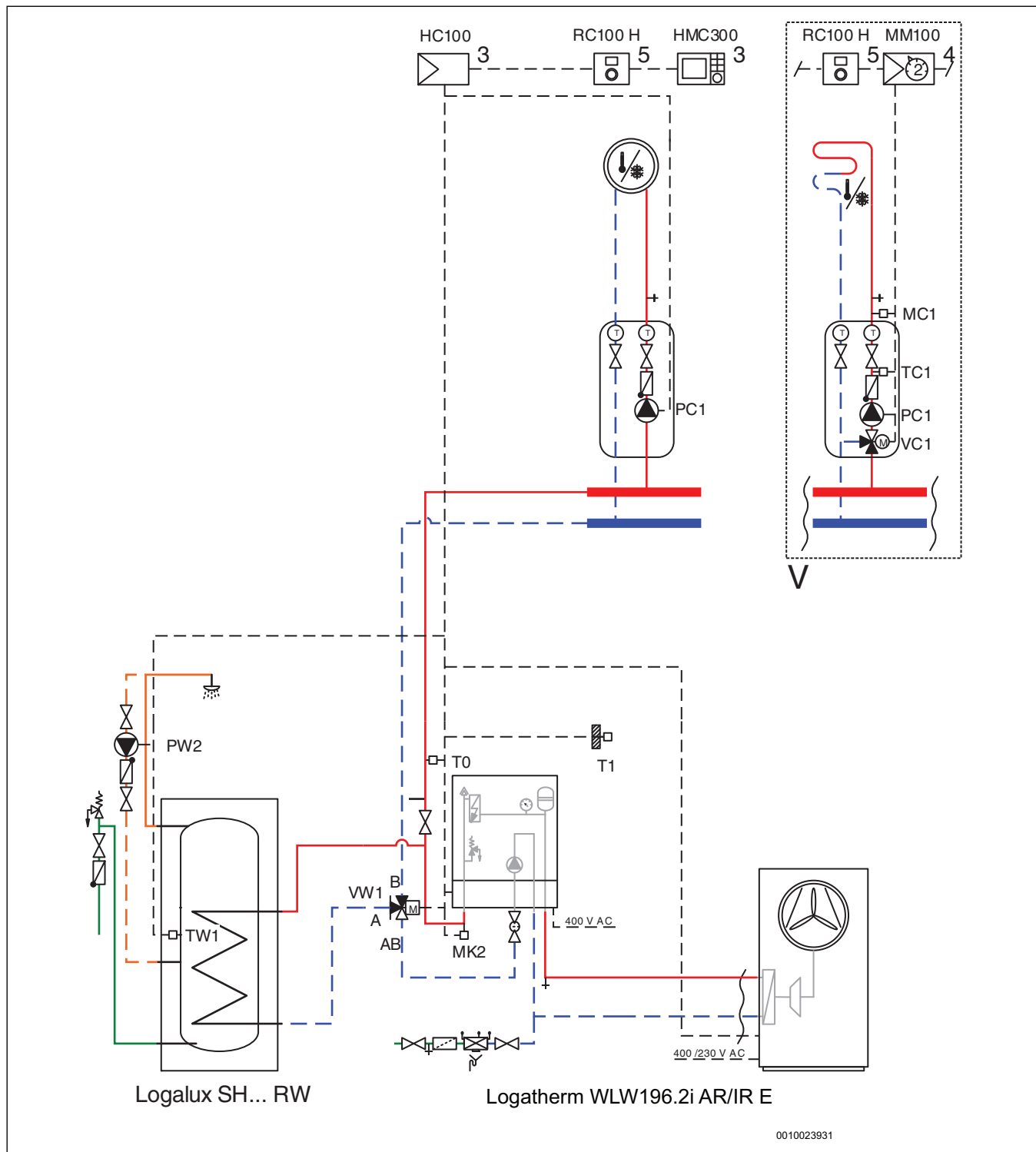
Bild 27 Elektrischer Zuheizter mit Warmwasserbereiter
