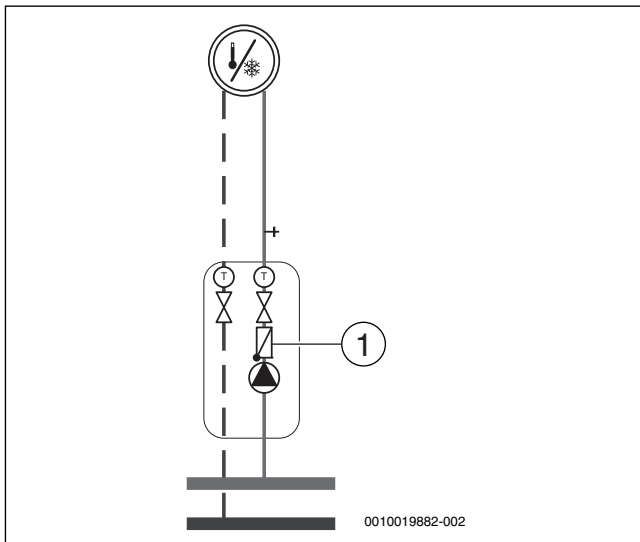
Bild 26 Heizkreis
