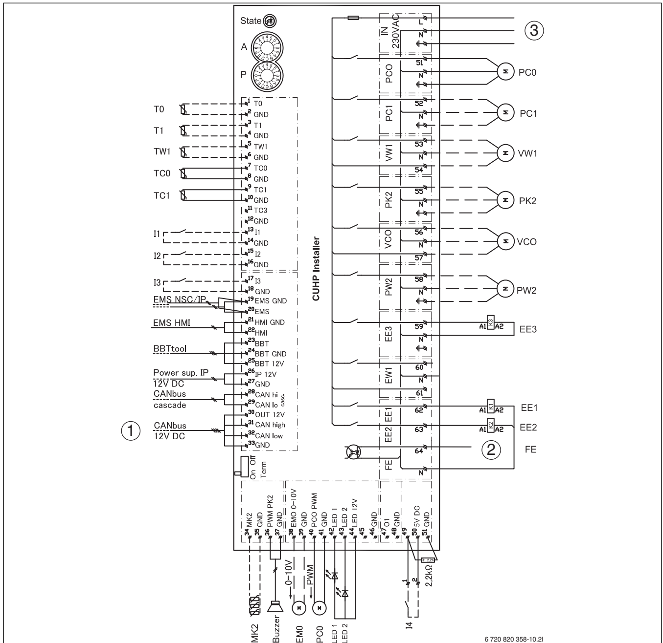
Bild 31 Schaltplan Installationsmodul mit integriertem elektrischen Zuheizier
