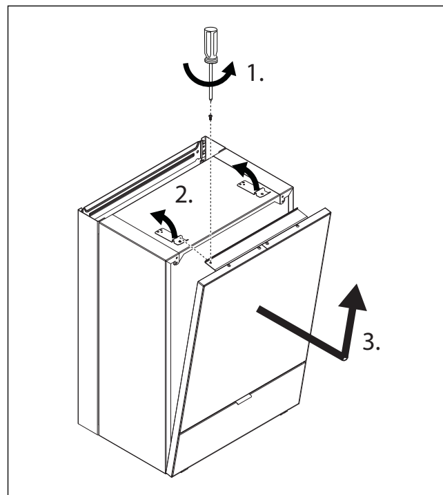
Bild 5 Frontplatte abnehmen
