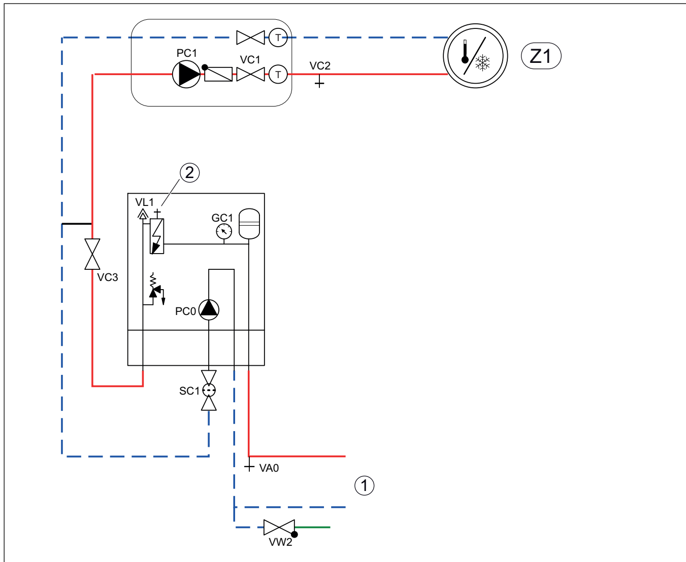
Bild 14 Inneneinheit mit integriertem elektrischem Zuheizter und Heizsystem
