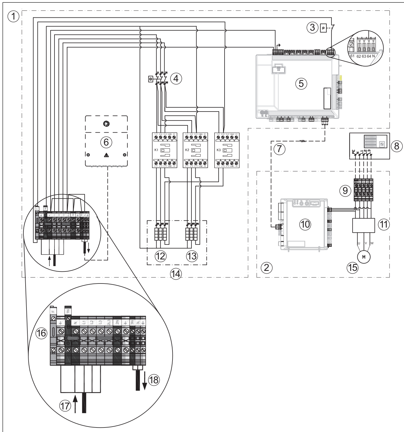
Bild 30 Wärmepumpe (Drehstrom) mit integriertem elektrischen Zuheizter (Drehstrom)
