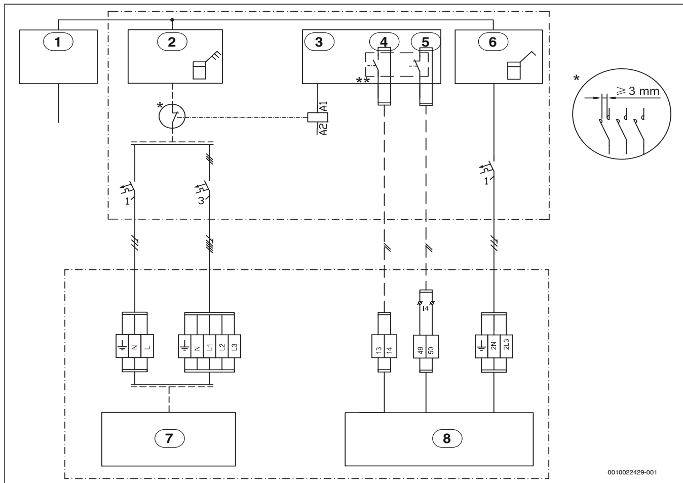
Bild 37 EVU Typ 2
