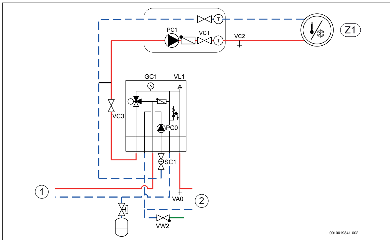
Bild 15 Inneneinheit mit externem Zuheizter und Heizsystem
