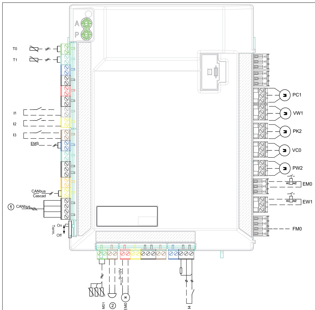
Bild 12 Anschlüsse Installationsmodul
