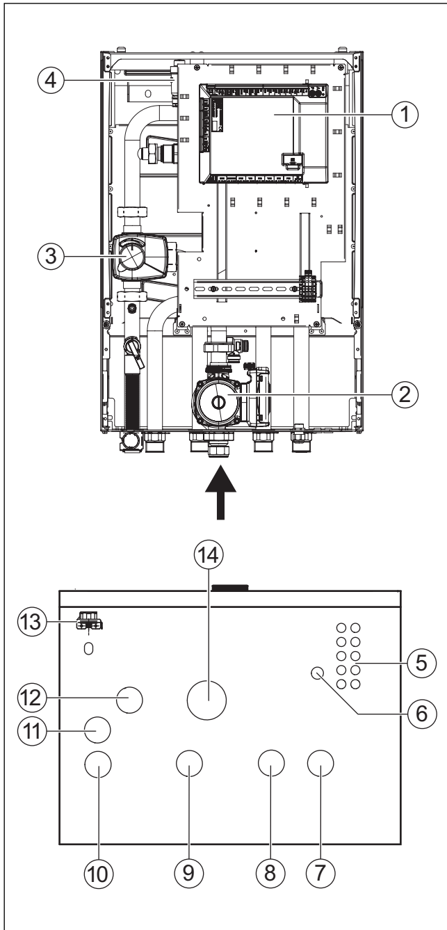
Bild 2 Bestandteile und Rohranschlüsse der Inneneinheit mit Mischer für externen Zuheizler
