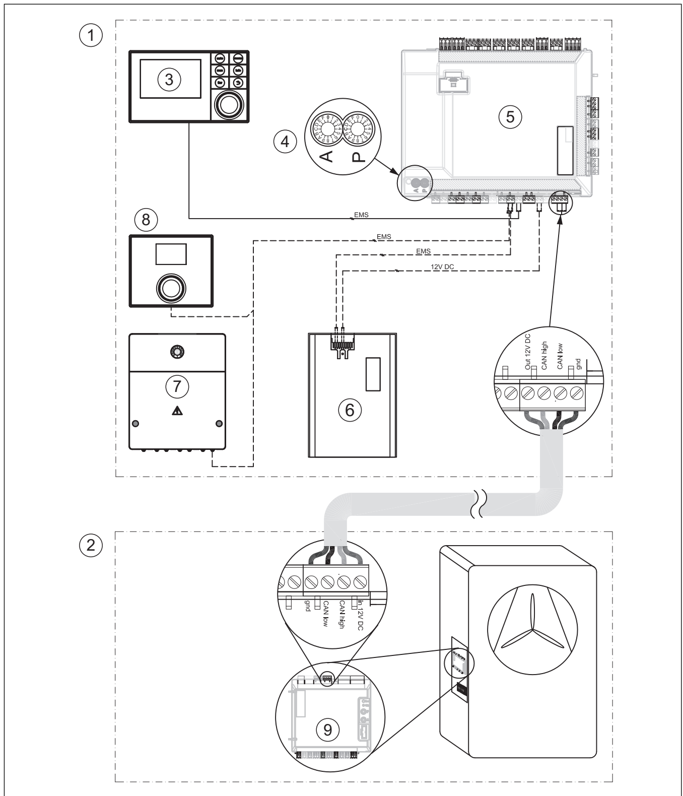
Bild 29 Inneneinheit mit Mischer für externen Zuheizter – Überblick CAN-/EMS-BUS
