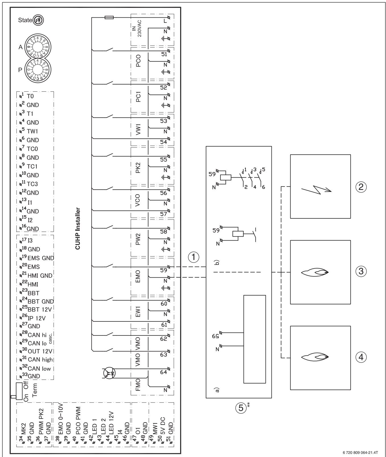
Bild 33 Schaltplan für Installationsmodul, Start/Stop mit externem Zuheizer
