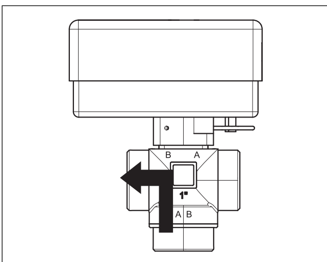
Bild 22 Kontakt offen, Anschluss B offen
