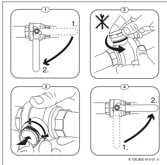
Bild 17 Siebreinigung
