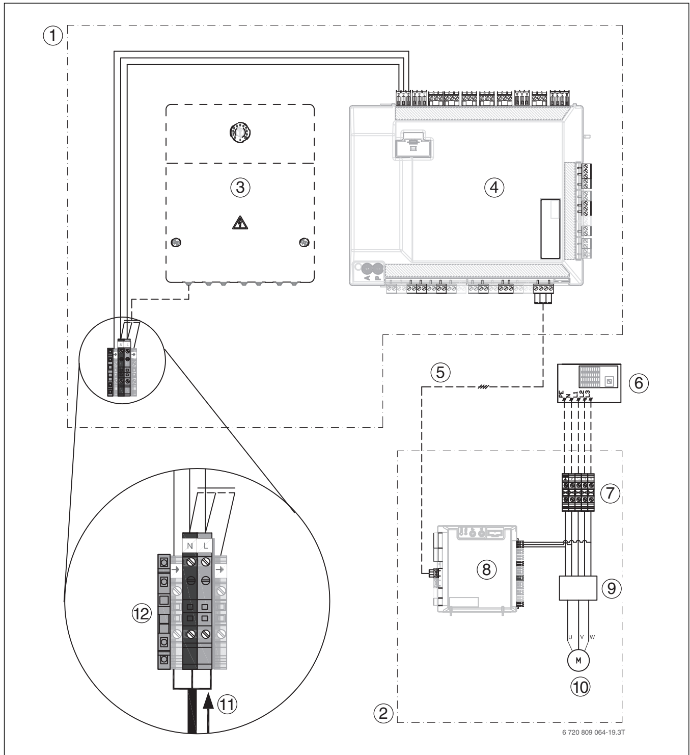
Bild 31 Dreiphasige Wärmepumpe und Inneneinheit mit externem Zuheizler
