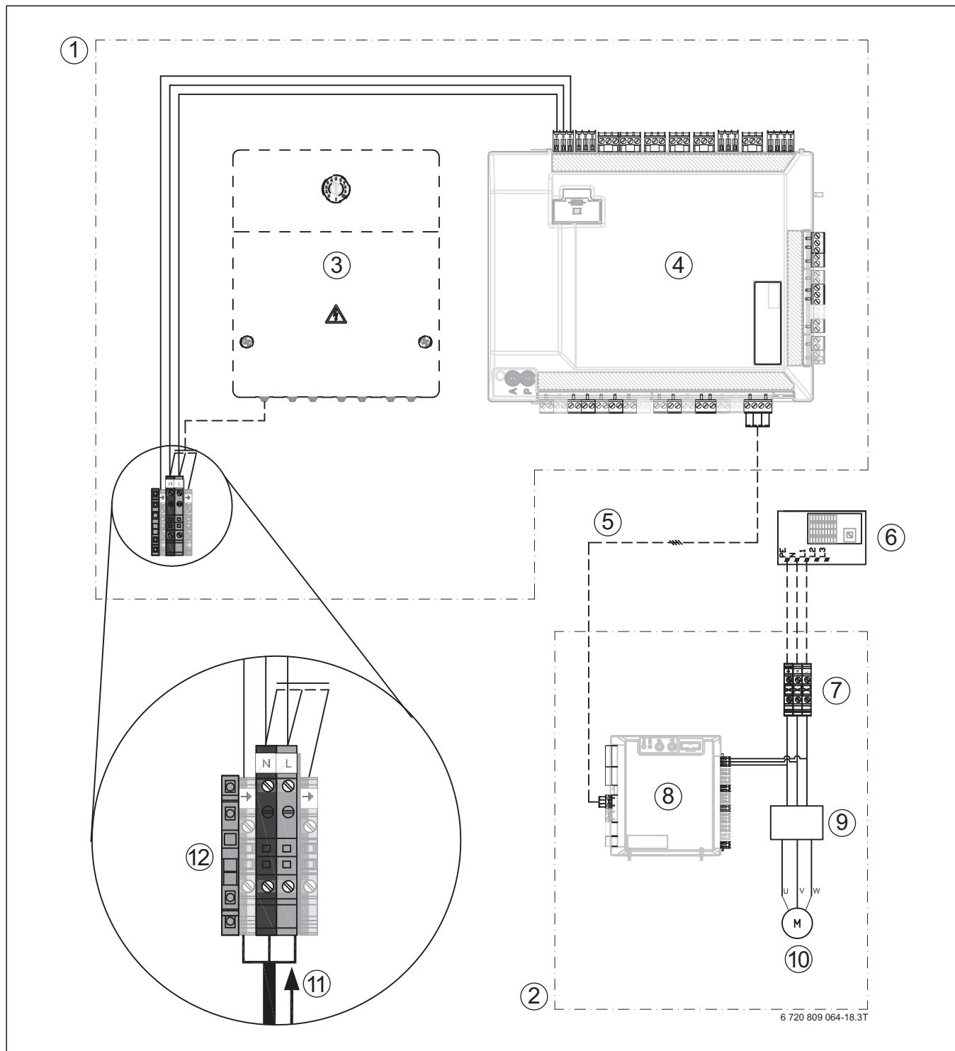
Bild 30 Einphasige Wärmepumpe und Inneneinheit mit externem Zuheizter
