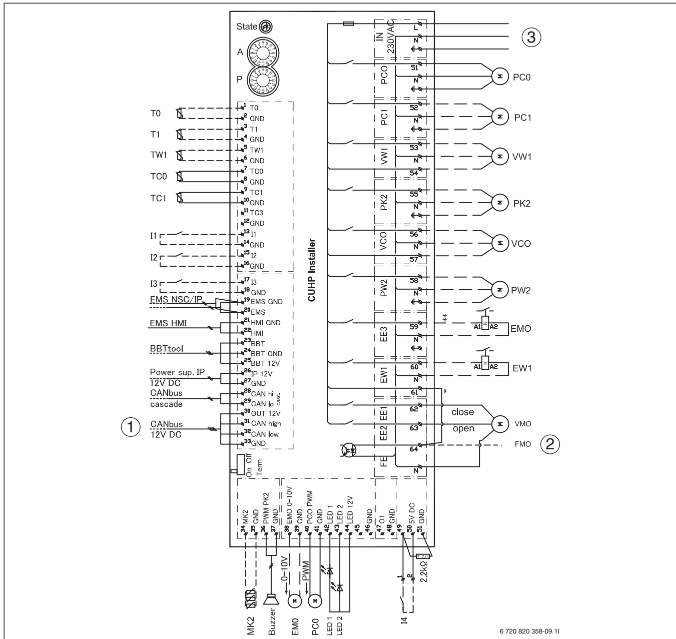
Bild 32 Schaltplan Installationsmodul für Inneneinheit mit Mischer für externen Zuheizier
