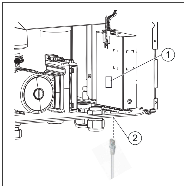
Bild 25 IP-Modul
