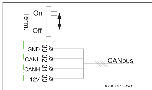
Bild 9 CAN-BUS-Terminierung
