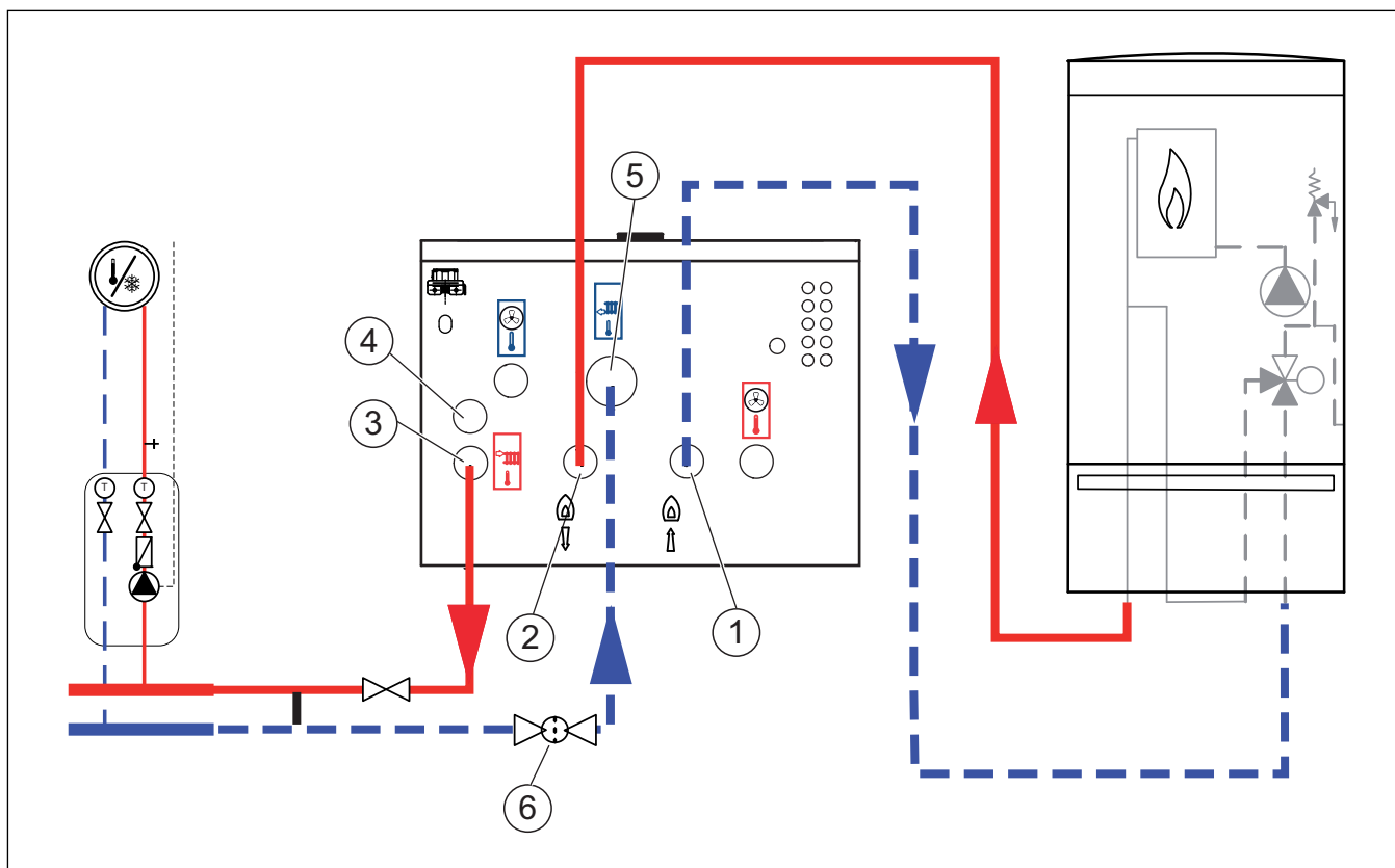
Bild 7 Anschluss der Inneneinheit mit Mischer für externen Zuheizier an die Heizungsanlage und den Zuheizier
