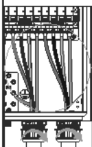
19 Schließen Sie Netz- und Verbraucherkabel an die entsprechenden Klemmen in der Matebox an.
