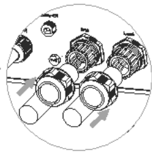
18 Führen Sie die Netz- und Verbraucherkabel durch den Netz- und Verbraucher-Port und dann in die Matebox.
