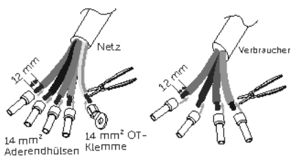
16 Die Kabel LL, L2, L3 und N 12 mm abisolieren.
