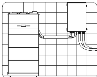
20 Verbinden Sie das Netzkabel mit dem Stromnetz und das Verbraucherkabel mit den Haushaltsverbrauchern.
