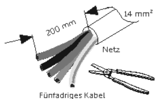
15 Netz- und Verbraucherkabel abisolieren.
