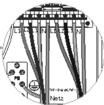
19 Schließen Sie Netz- und Verbraucherkabel an die entsprechenden Klemmen in der Matebox an.
