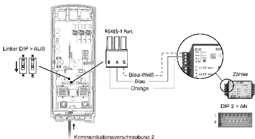
Abbildung 16: Anschluss des Zählers 2
