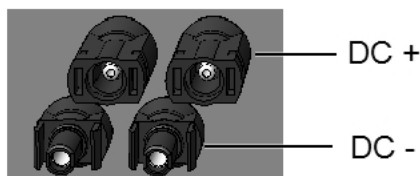
Abbildung 14: Wechselrichter DC-Anschlüsse
