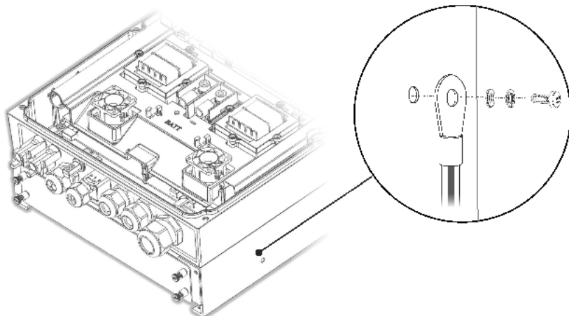
Abbildung 20: Erdung der Batterie
