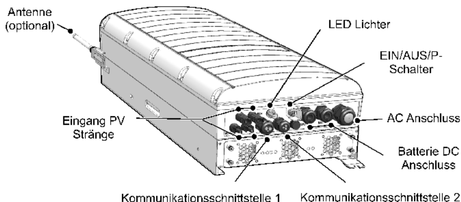
Abbildung 5: Wechselrichterschnittstellen
