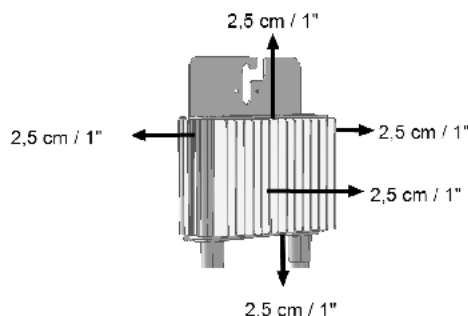
Abbildung 2: Abstand bei Leistungsoptimierern
