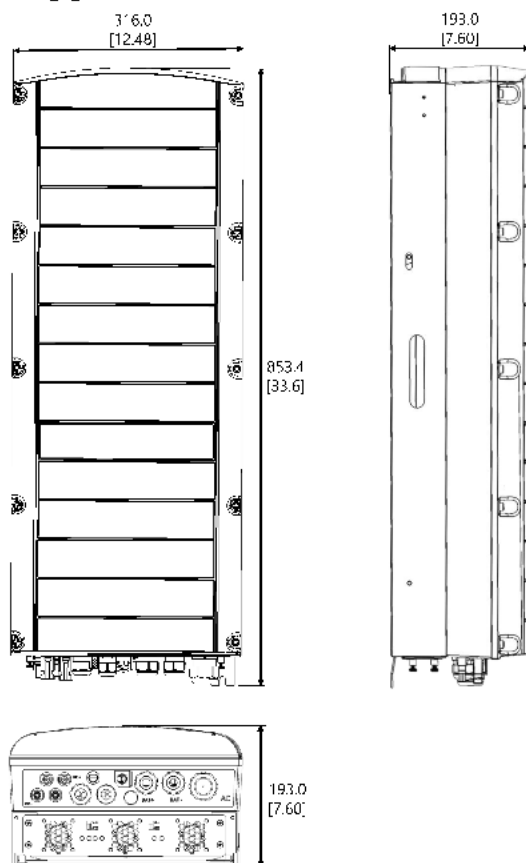
Abbildung 21: Maße des StorEdge Dreiphasen-Wechselrichters:
