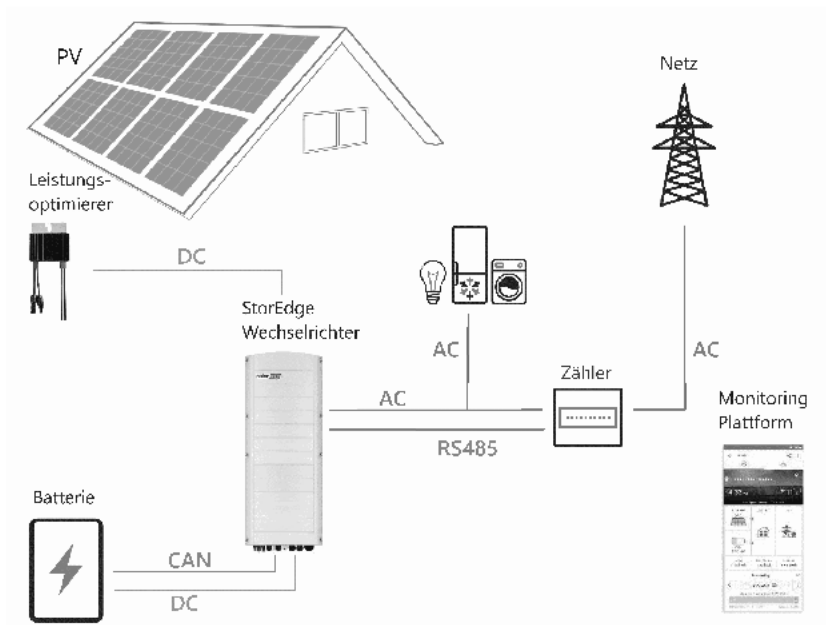
Abbildung 1: StorEdge Systemkomponenten
