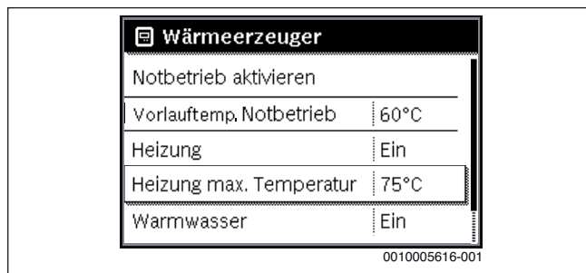
Bild 44 Maximale Vorlauftemperatur
