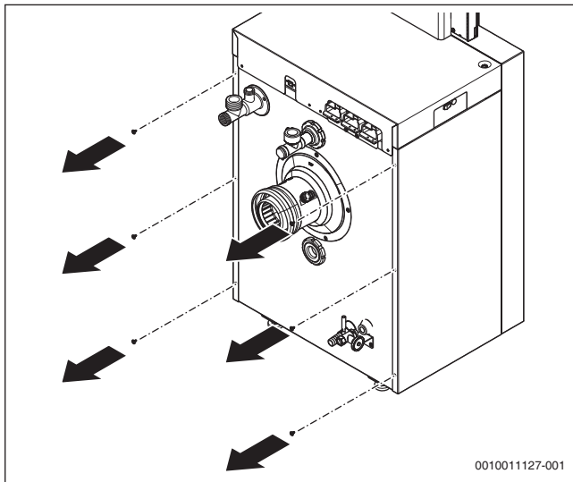
Bild 83 Befestigungsschrauben lösen
