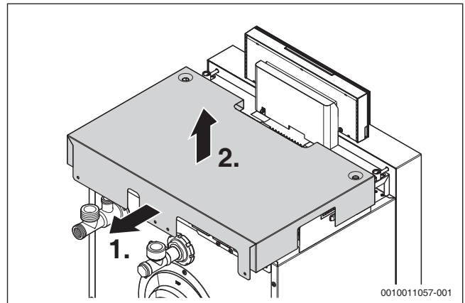
Bild 21 Kesselhaube abnehmen
