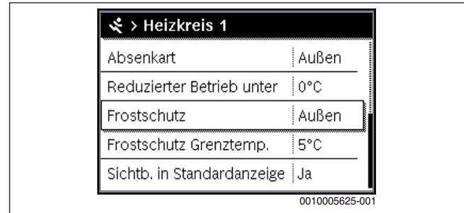
Bild 49 Frostschutz einstellen
