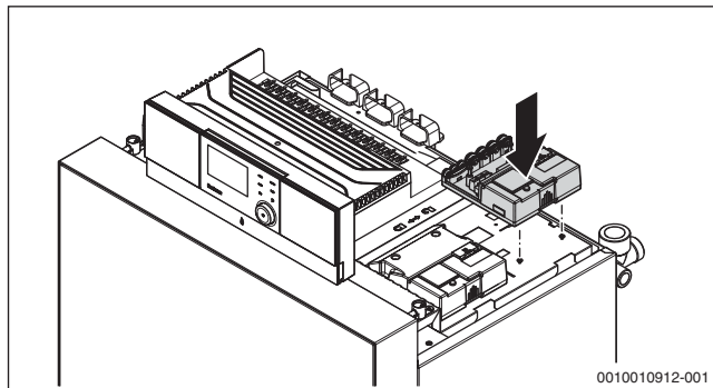
Bild 32 Funktionsmodul aufsetzen
