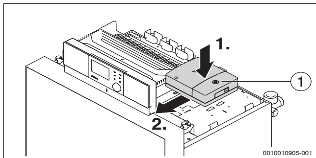
Bild 27 Funktionsmodule einstecken
