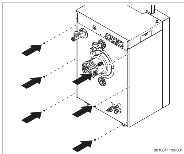
Bild 89 Seitenwände befestigen
