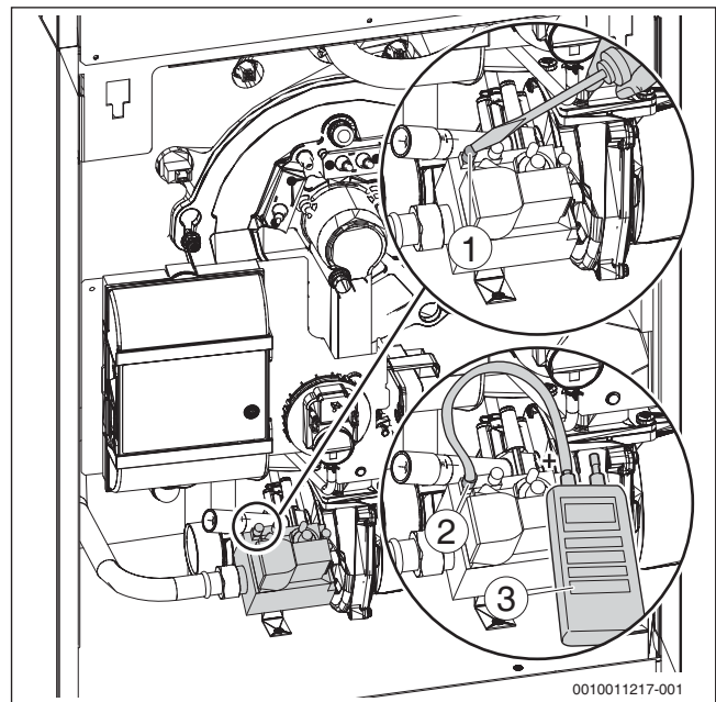
Bild 68 Gas-Anschlussdruck messen
