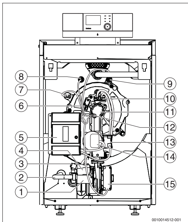
Bild 101 Vorderansicht
