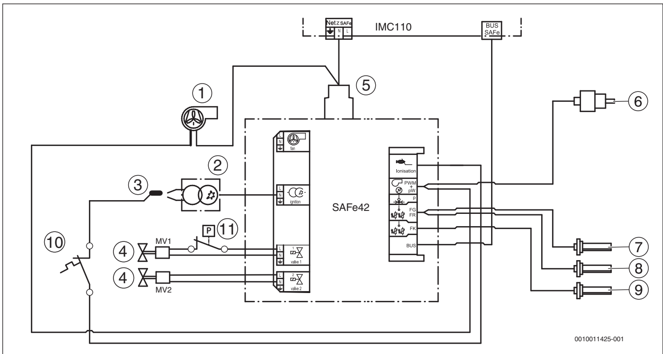
Bild 100 Anschlussplan Feuerungsautomat (50 kW)
