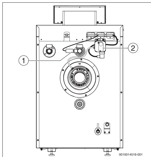
Bild 102 Rückansicht
