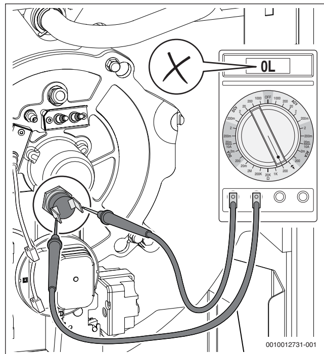
Bild 95 Elektrischen Widerstand an den Kontakten des Temperaturwächters messen (Temperaturwächter nicht in Ordnung)
