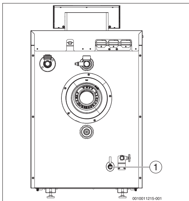
Bild 14 Kondensatschlauch montieren
