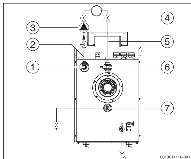
Bild 15 Anschlussschema Hydraulik
