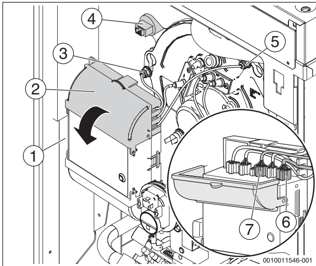
Bild 71 Steckverbinder lösen
