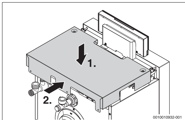
Bild 24 Kesselhaube montieren
