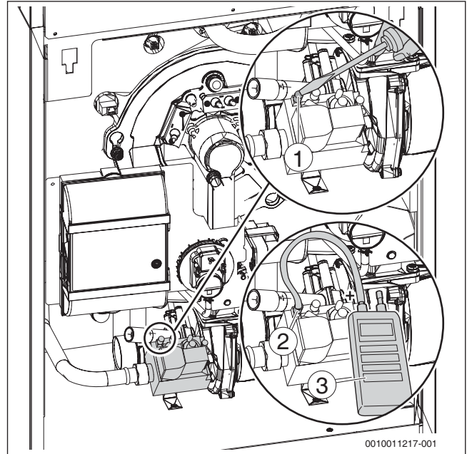
Bild 53 Gas-Anschlussdruck messen
