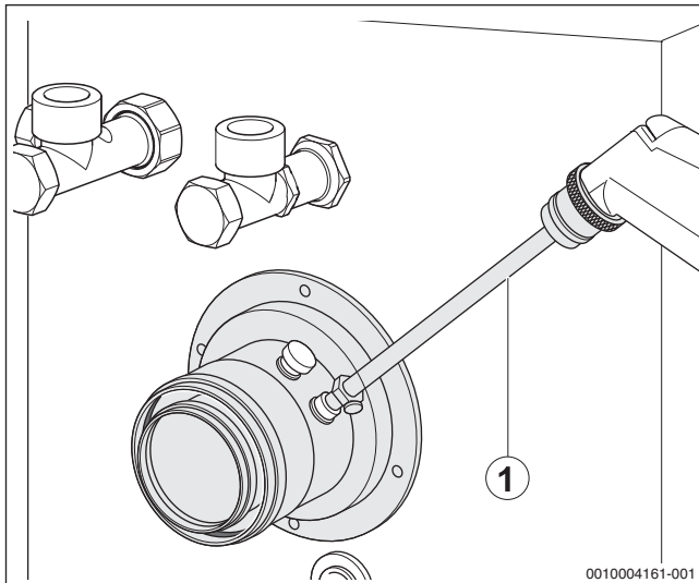
Bild 57 Messwerte aufnehmen
