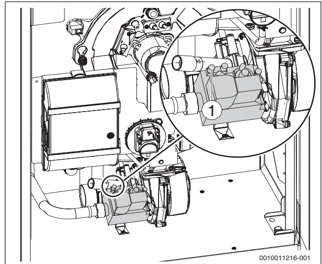
Bild 36 Gasleitung entlüften
