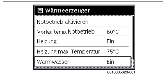
Bild 46 Warmwasserbereitung einschalten
