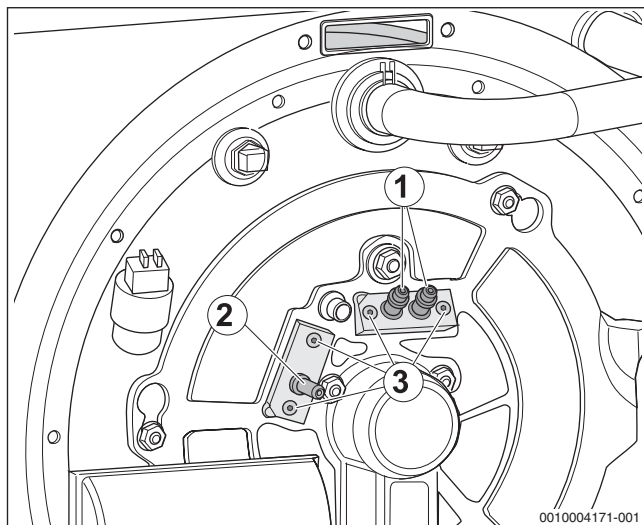
Bild 80 Elektrodenposition
