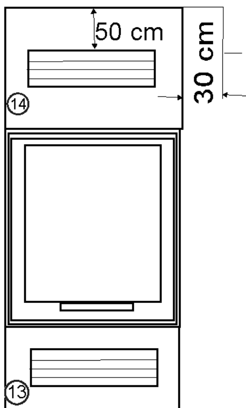
Abb. 8: Konvektionsführung
