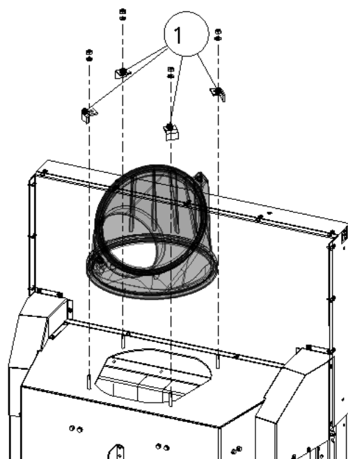
Abb. 34: Rauchsammler abmontieren
