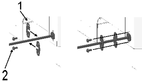
Abb. 51: Flansch Bowdenzug
