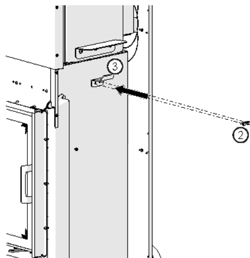
Abb. 25: HMS-Halter montieren
