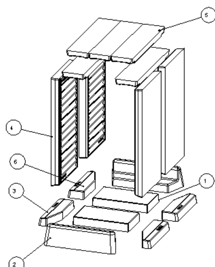
Abb. 20: Keramott 45x51 KII
