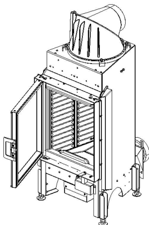
Abb. 72: Tür öffnen
