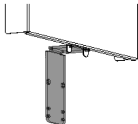
Abb. 61: KV-Wand rechts und links einrasten
