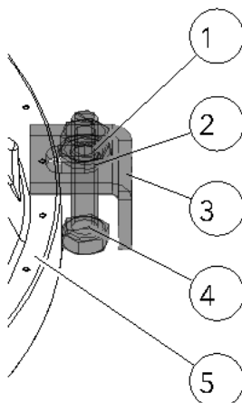
Abb. 36: Abgassammler montieren
