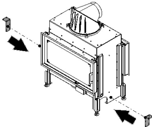
Abb. 64: Halterung links und rechts montieren
