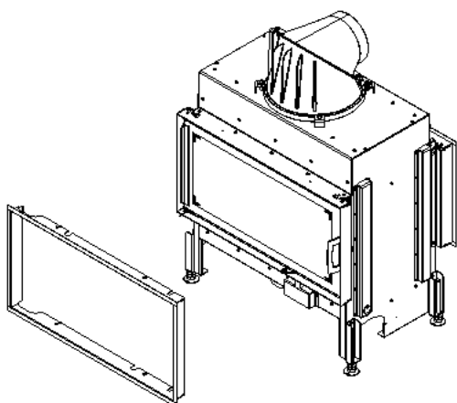
Abb. 80: Designrahmen positionieren
