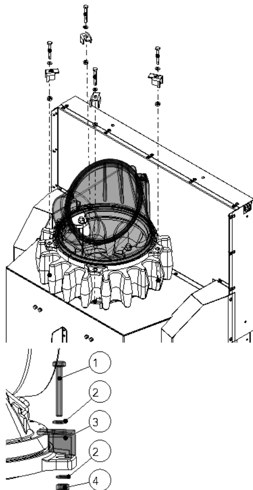
Abb. 33: Rauchsammler montieren
