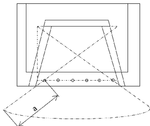
Abb. 12: a: Sicherheitsabstand
