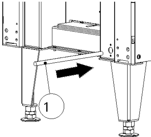
Abb. 48: Bowdenzug einfädeln
