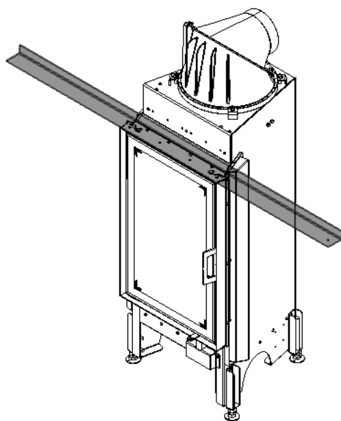
Abb. 87: Tragrahmen montieren
