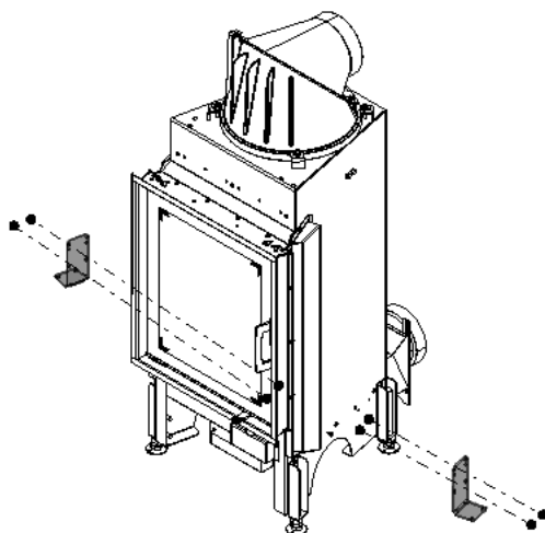
Abb. 54: Halterung links und rechts montieren
