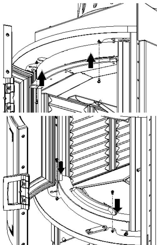
Abb. 79: Designrahmen befestigen
