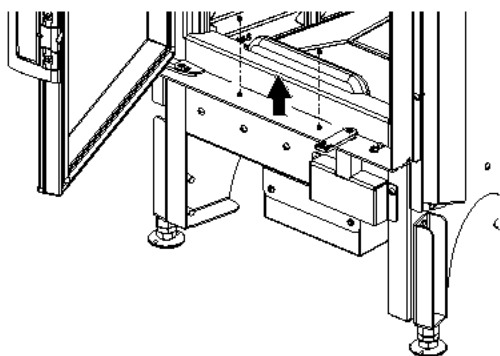
Abb. 74: Bolzen unten rausdrehen
