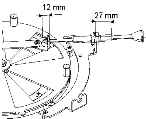
Abb. 49: Bowdenzug verbinden
