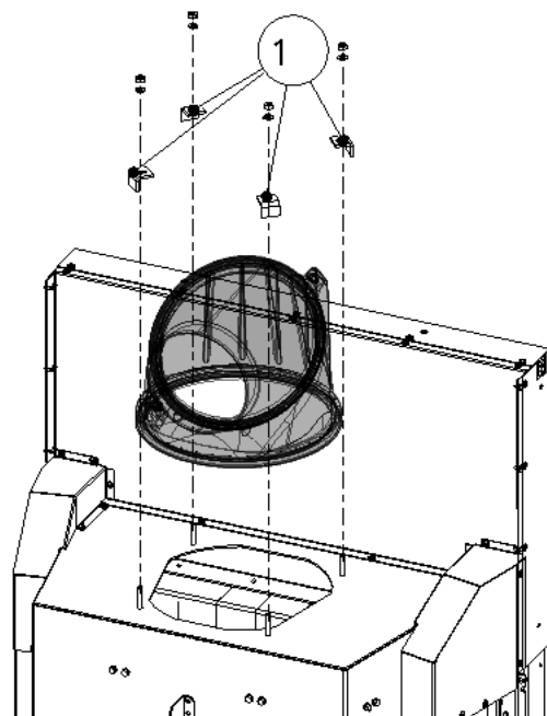
Abb. 27: Rauchsammler abmontieren
