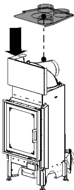
Abb. 59: KV-Deckel montieren
