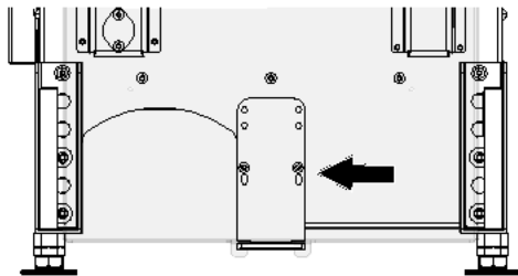
Abb. 66: KVM 75x39 KII
