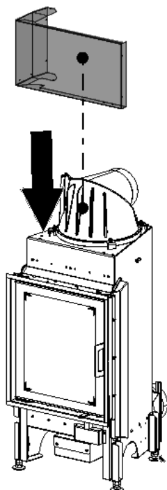
Abb. 58: KV-Wand vorne montieren
