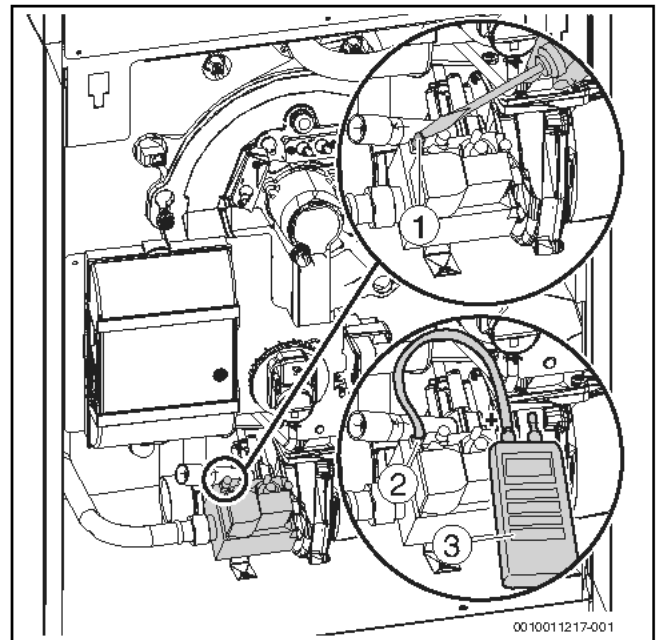
Bild 53 Gas-Anschlussdruck messen
