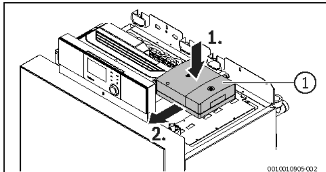
Bild 27 Funktionsmodule einstecken
