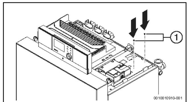
Bild 32 Schrauben eindrehen
