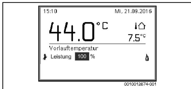
Bild 50 Abgastestbetrieb aktiv
