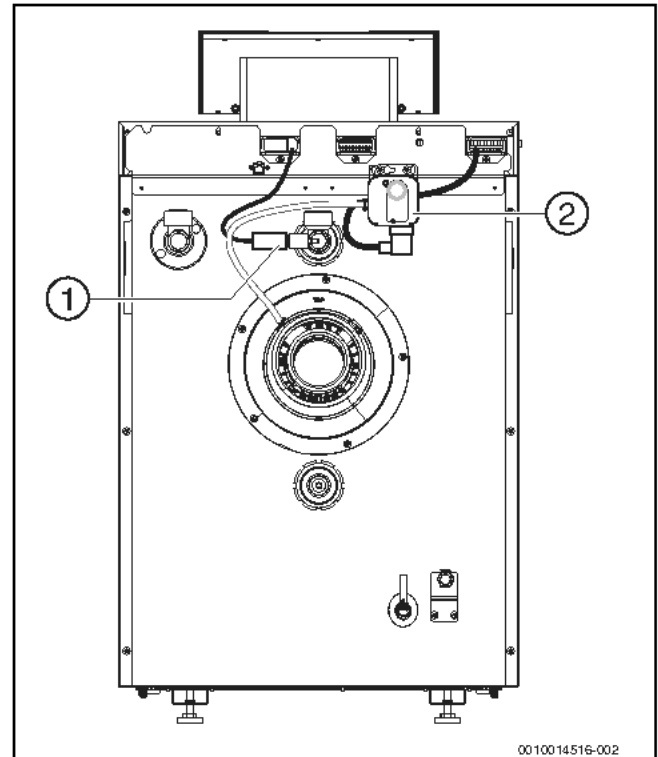
Bild 103 Rückansicht
