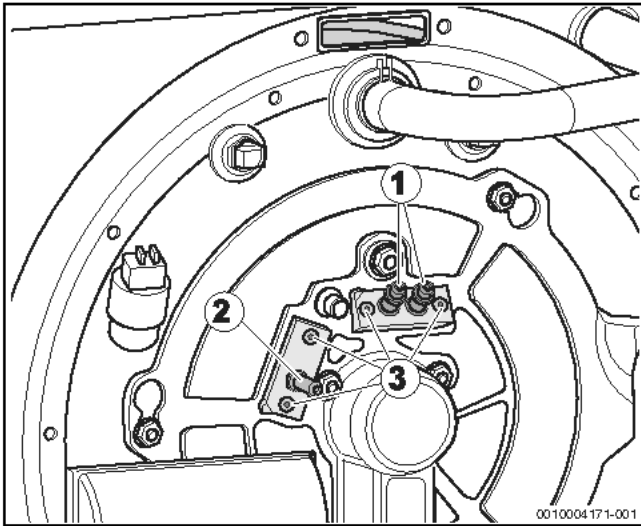
Bild 80 Elektrodenposition
