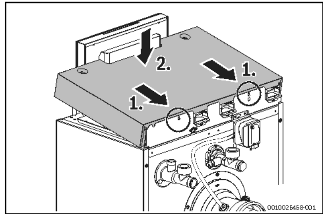
Bild 25 Kesselhaube montieren
