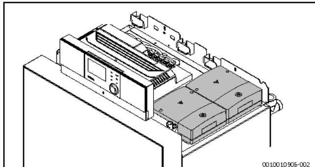
Bild 28 Standard-Funktionsmodule montiert
