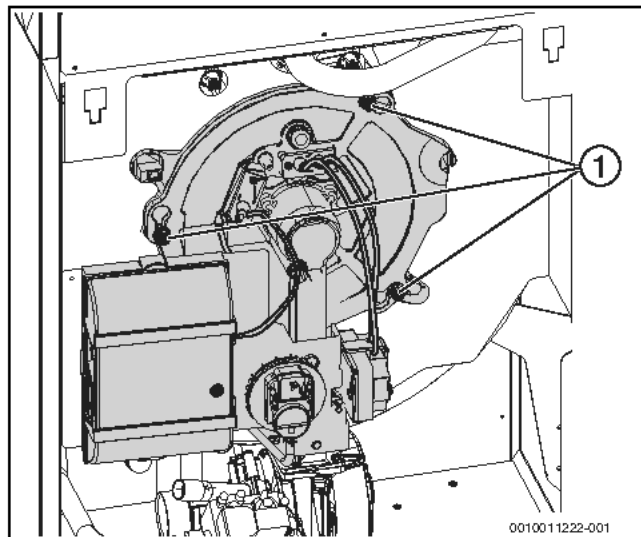
Bild 75 Befestigungsmutter lösen
