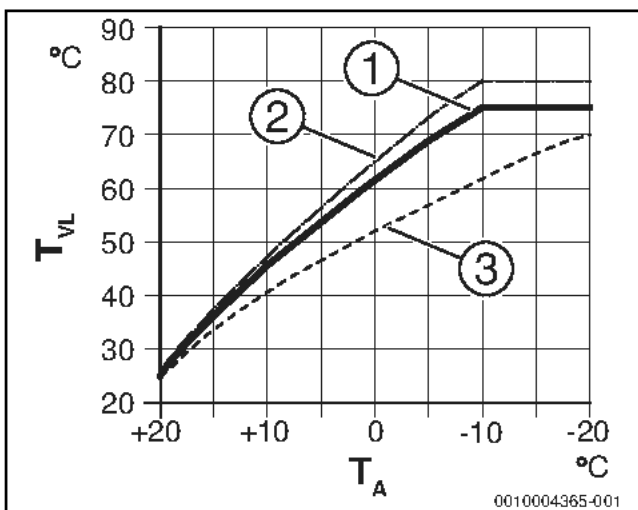
Bild 63 Einstellung der Heizkurve für Heizkörper Steigung über Auslegungstemperatur T_{AL} und minimale Außentemperatur T_{A,\min}
