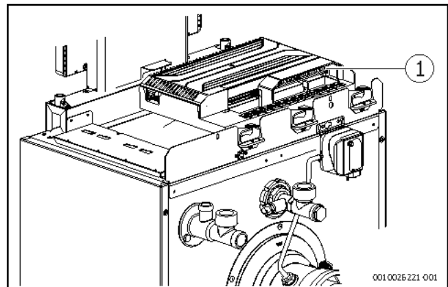
Bild 26 Netzanschluss herstellen
