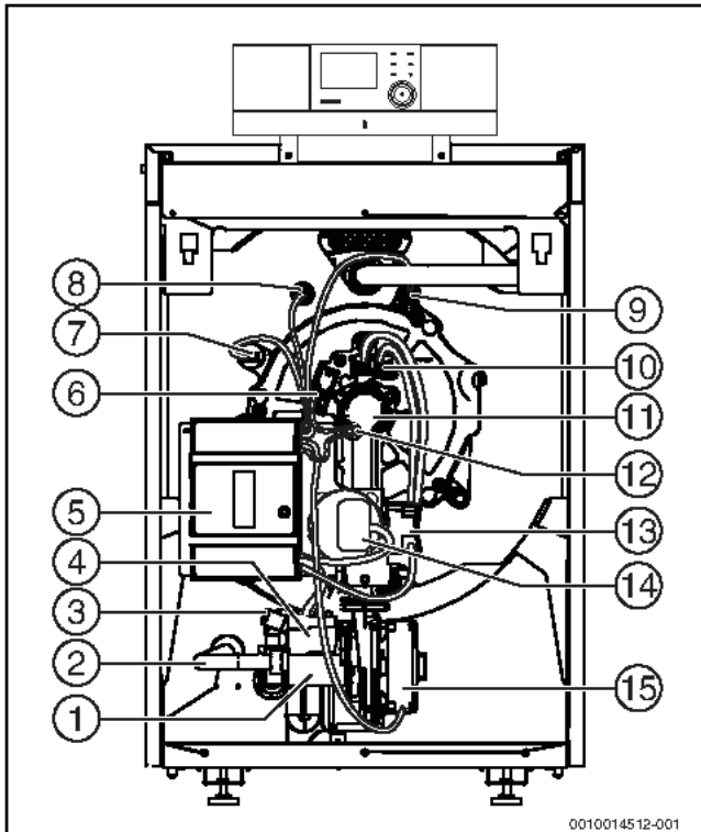
Bild 102 Vorderansicht
