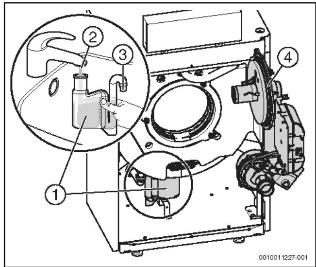
Bild 82 Siphon reinigen
