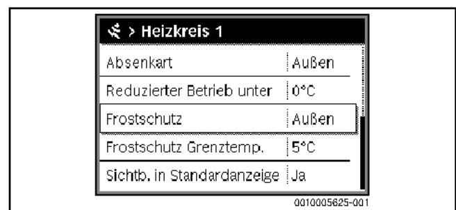
Bild 49 Frostschutz einstellen
