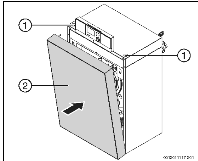
Bild 59 Kesselvorderwand montieren
