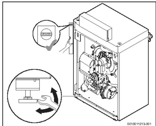
Bild 10 Heizkessel ausrichten
