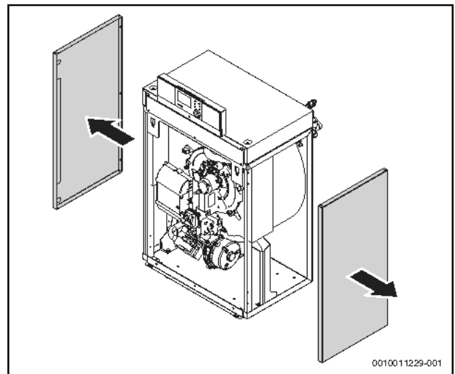
Bild 86 Seitenwände abnehmen
