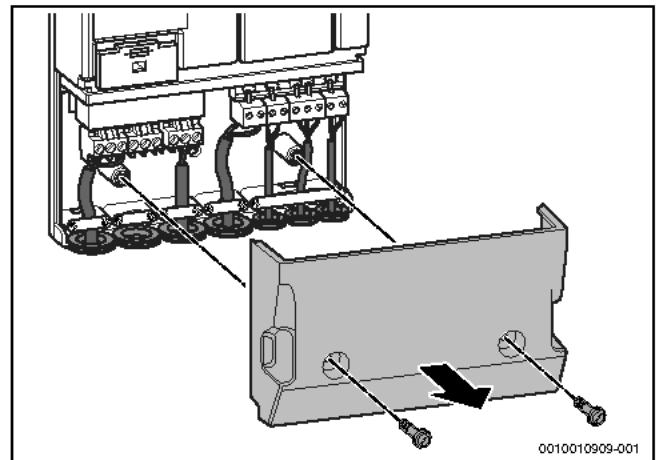
Bild 31 Funktionsmodul öffnen
