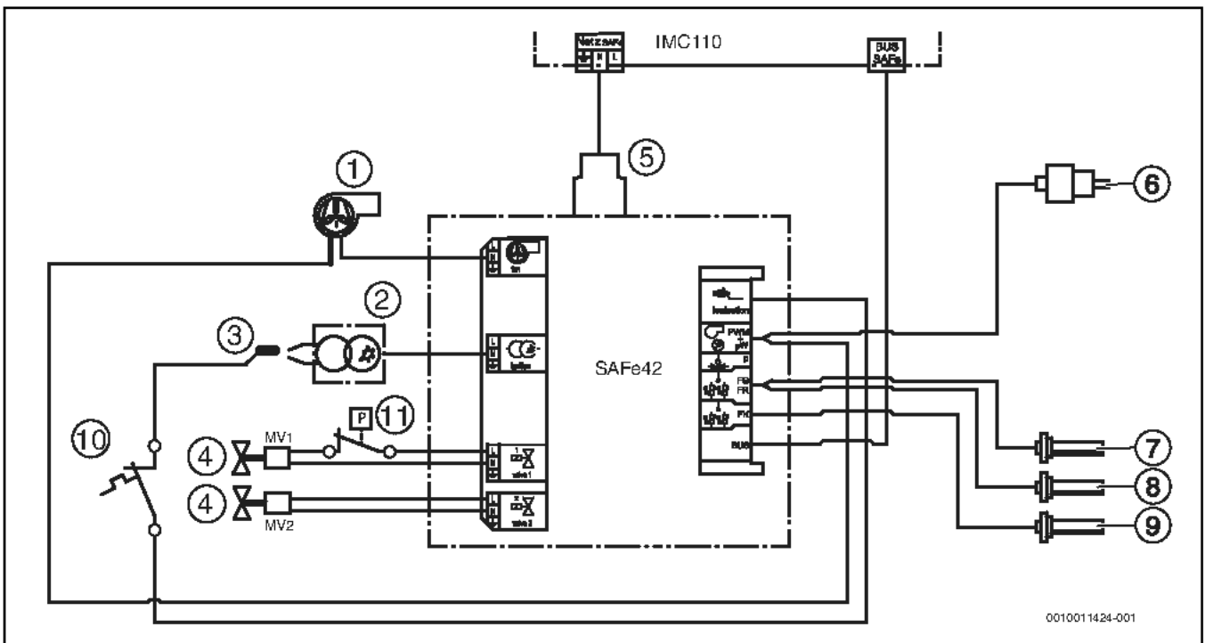
Bild 100 Anschlussplan Feuerungsautomat (15...30 kW; auch 40 und 50 kW bei manchen Modellen)
