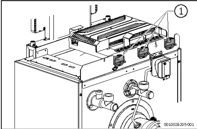
Bild 22 Kabel verlegen
