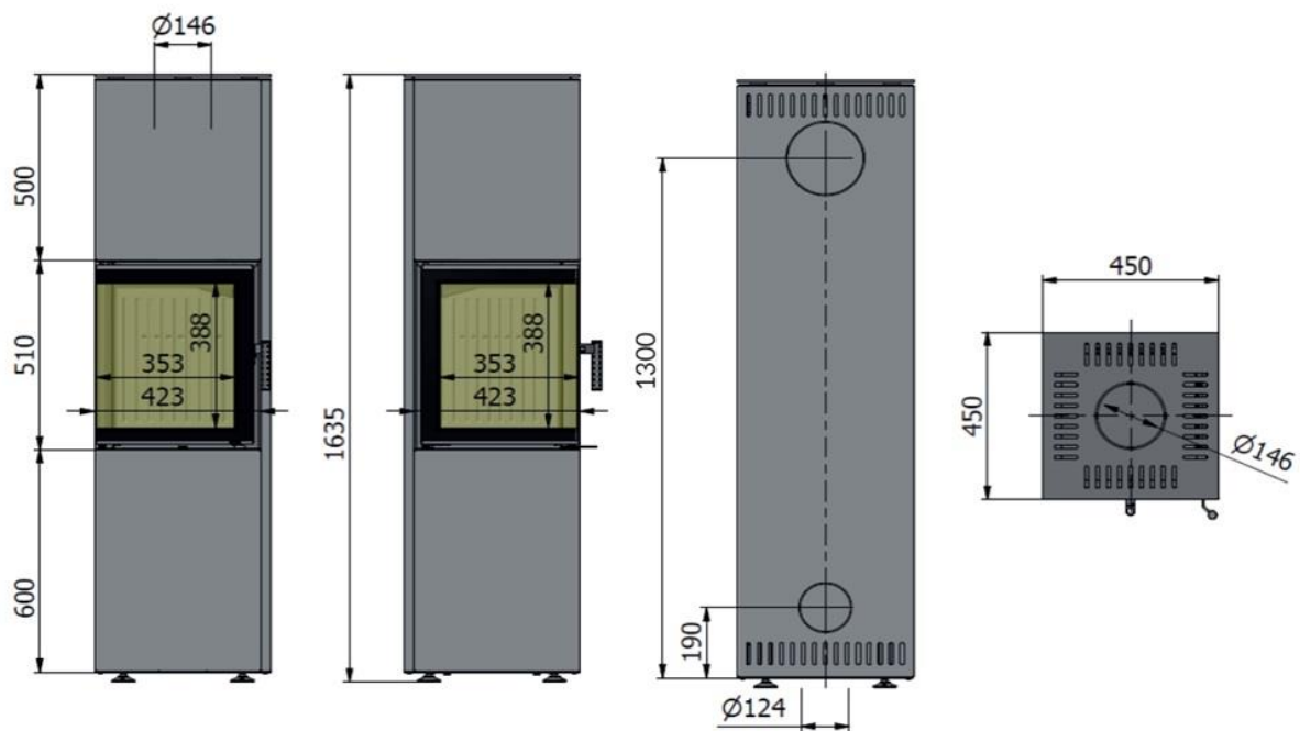
Abb.. 5. Maße des Kaminofens Pixel XL
