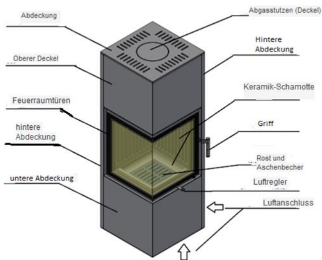
Abb. 1. Heizungsdesign– Beispiel PIXEL L
