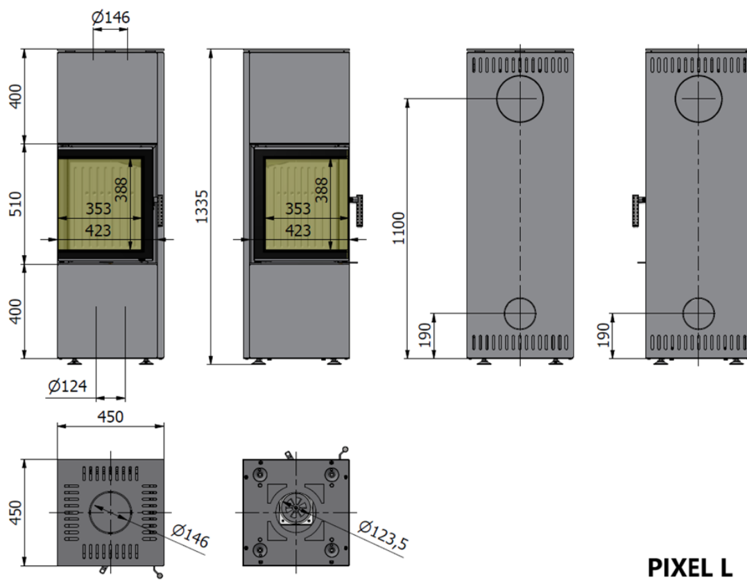
Abb.. 4. Maße des Kaminofens PIXEL L
