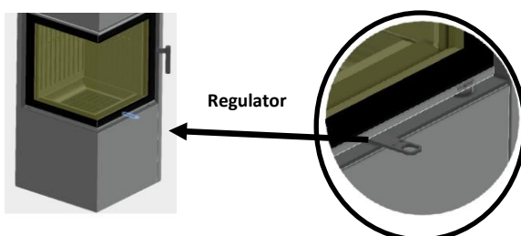
Abb. 13 Position des Luftreglers
