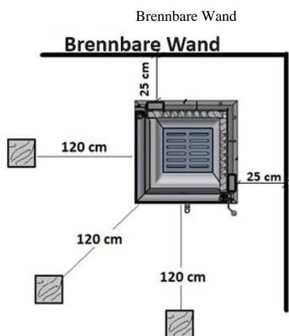
Abb.. 7. Notwendige Abstände zu brennbaren Elementen
