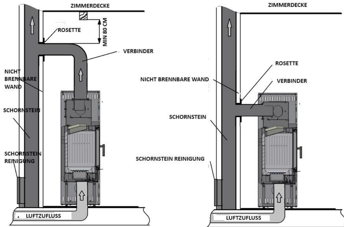
Abb.. 11. Verfahren zur Installation des Abgasanschlusses.
