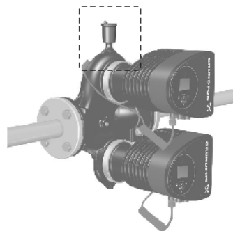
Automatischer Schnellentlüfter
