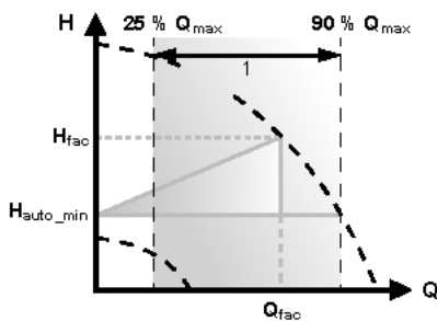
„FLOWADAPT“-Regelung
