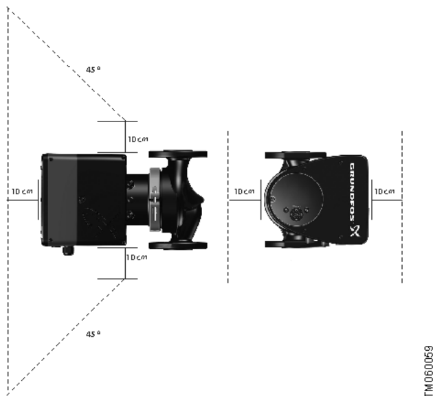
Mindestabstand um die Einzelpumpe
