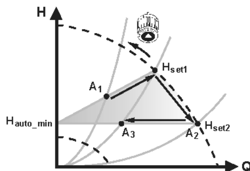
„AUTOADAPT“-Regelung
