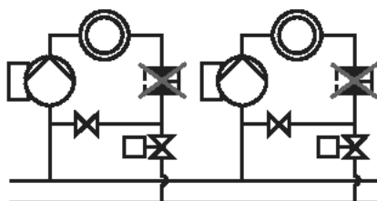
Einsparen von Drosselventilen
