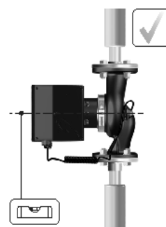
Pumpe mit Schaltkasten in horizontaler Position
