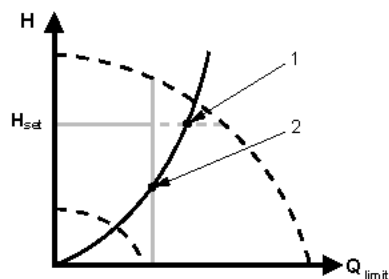
Konstantdruckregelung mit FLOW_{LIMIT}
