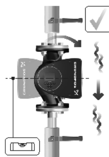
Pumpe mit Schaltkasten in horizontaler Position
