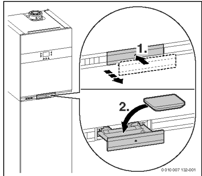
Bild 232 Heizungsregler einstecken
