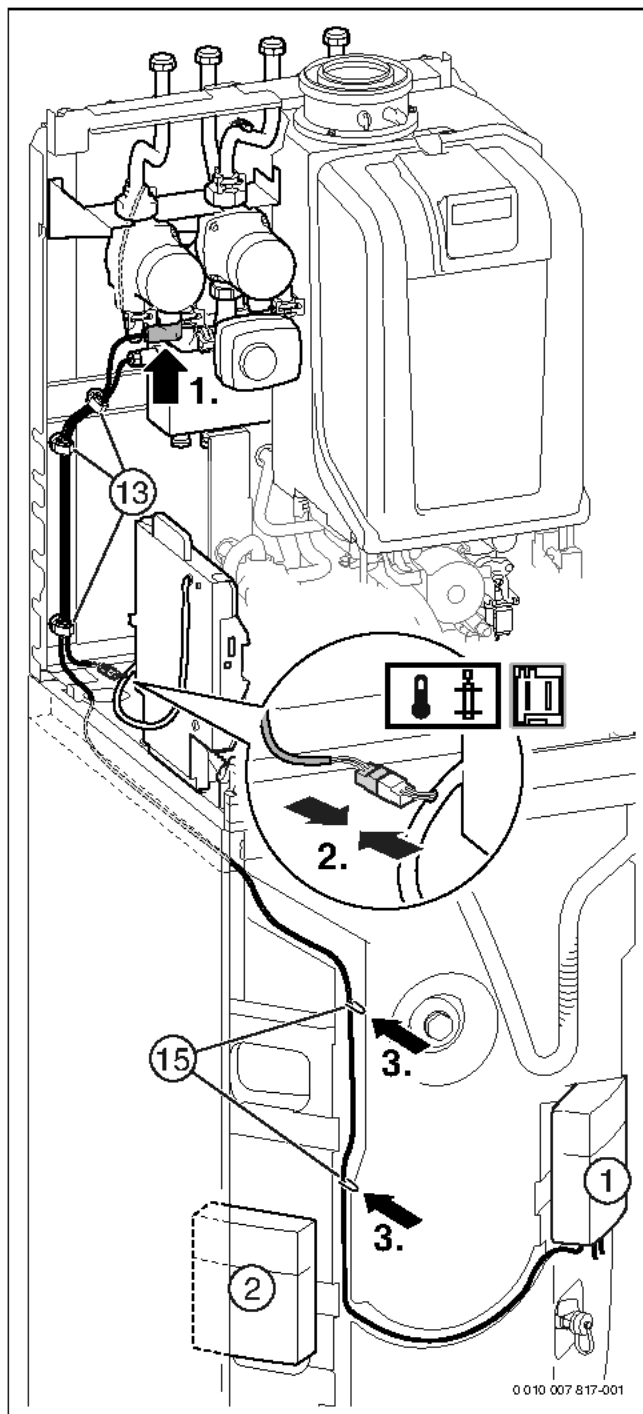
Bild 139 GB.192...iT150...Geräte: Anschluss Heizungspumpe ungemischter Heizkreis und Hydraulische Weiche
