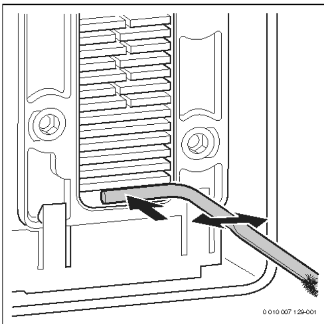
Bild 259 Kondensatwanne reinigen
