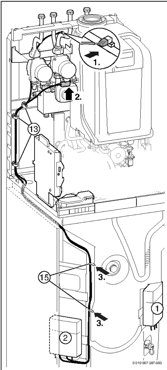
Bild 141 GB.192...iT150...-Geräte: Anschluss Heizungspumpe gemischter Heizkreis und Temperaturfühler
