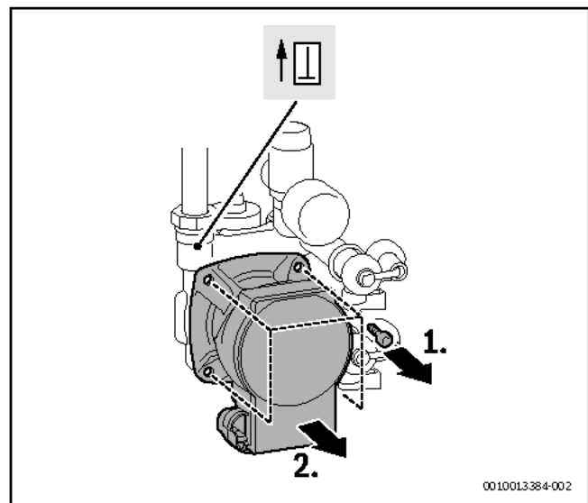
Bild 269 Solarpumpe ausbauen
