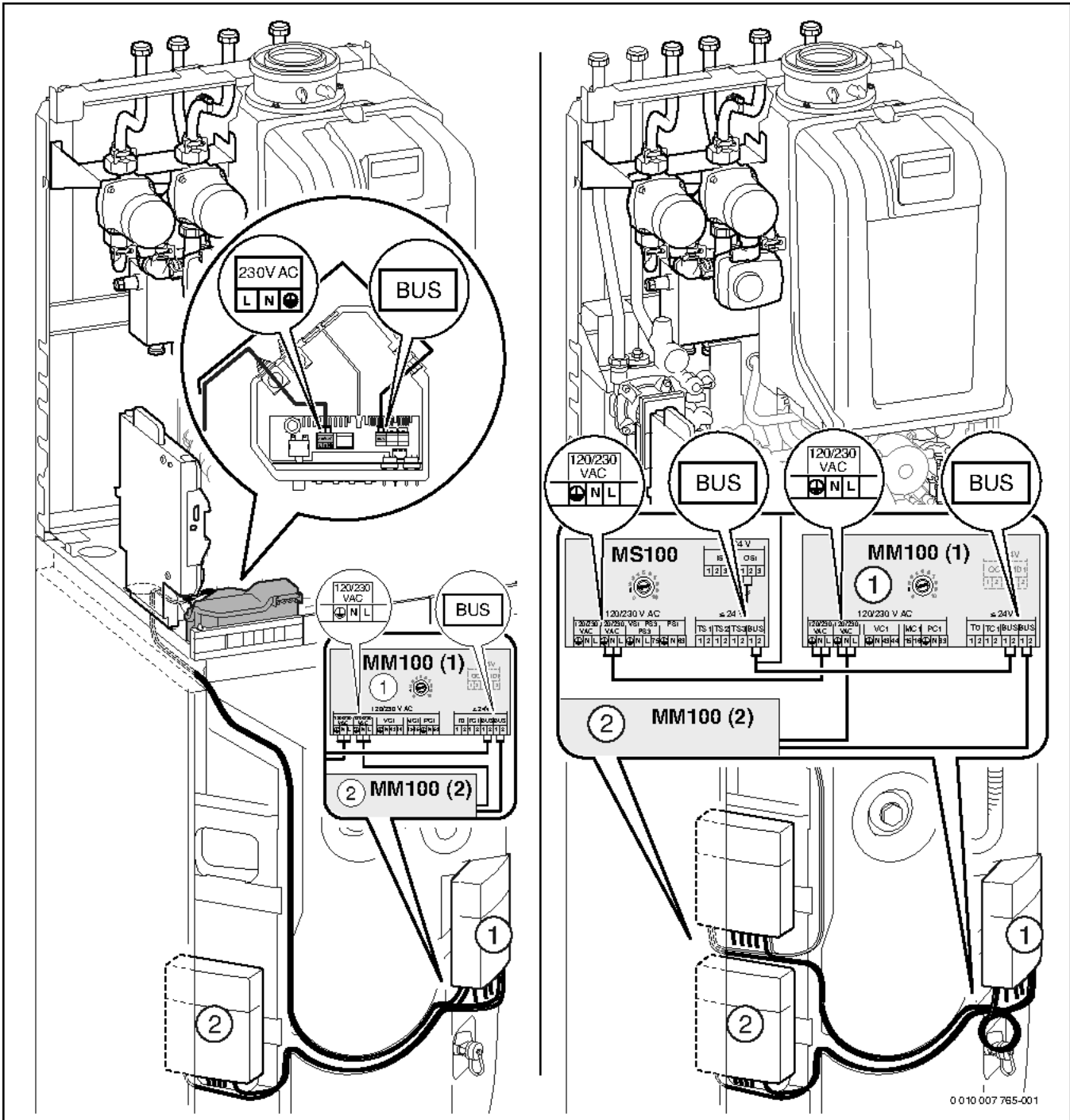
Bild 147 GB.192-...iT150.-Geräte: Anschluss ohne Modul MS100 (links) und mit Modul MS100 (rechts) durchschleifen
