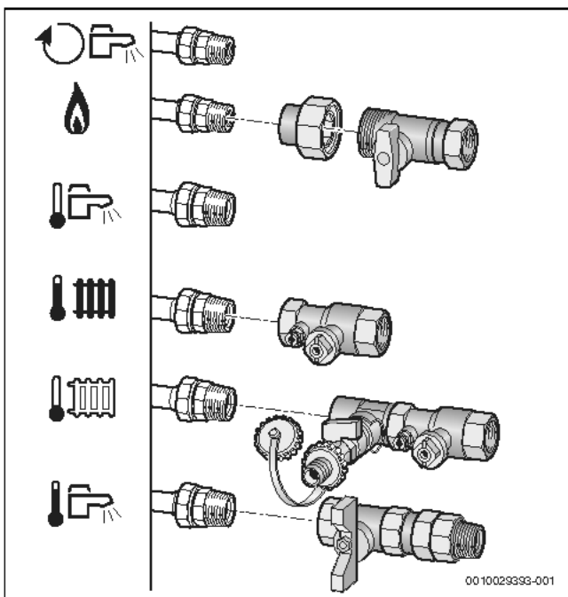
Bild 49 Montage des Armaturen-Sets am Beispiel Anschlüsse nach rechts AS-H1/Horizontales Anschluss-Set
