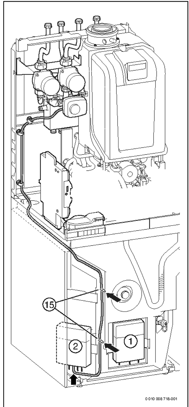
Bild 144 GB.192...iT100...-Geräte: Anschluss Mischermotor
