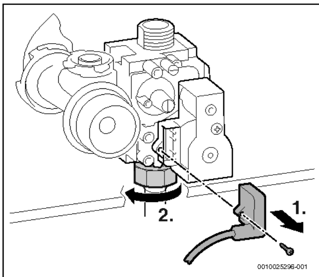
Bild 267 Stecker abziehen und Überwurfmutter lösen
