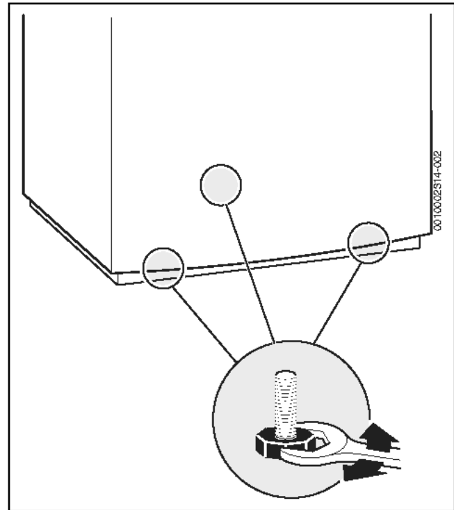
Bild 53 Speicher ausrichten
