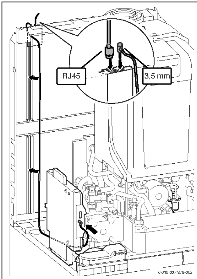
Bild 231 Anschluss und Verlegung des Kabels an Buderus Logamatic web KM100
