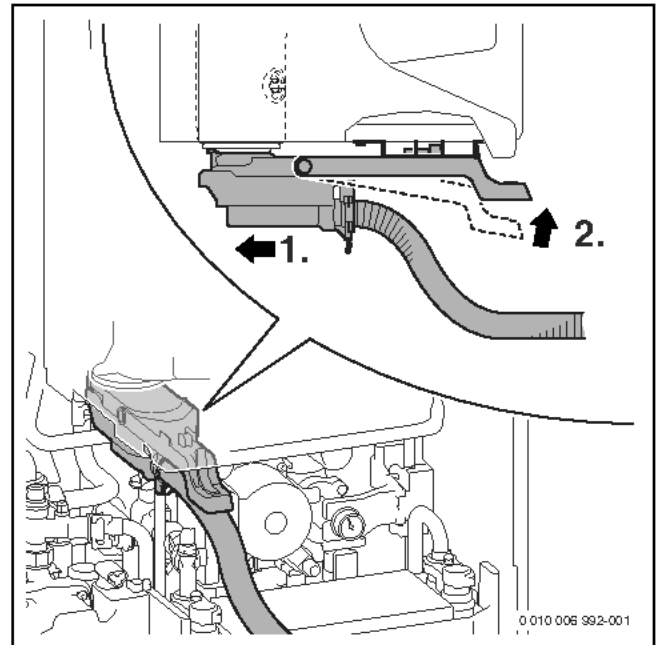
Bild 57 Schmutzfänger montieren
