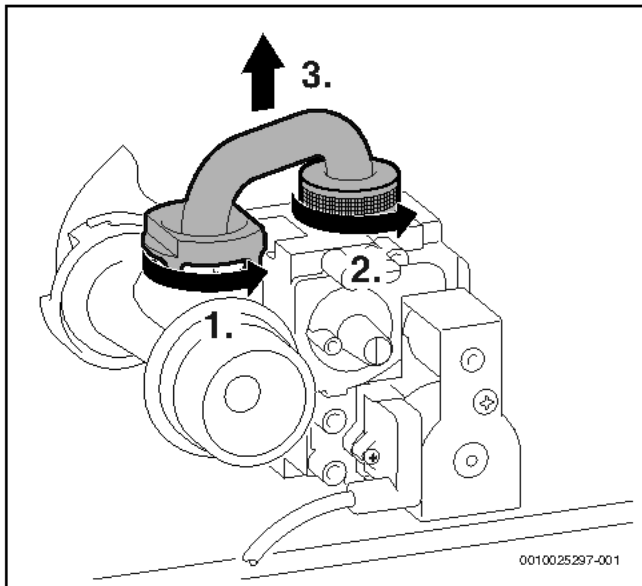
Bild 266 Gasrohr ausbauen
