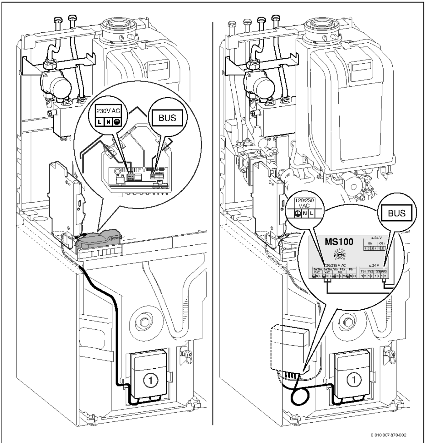
Bild 114 GB.192-...iT100...-Geräte: Anschluss ohne Modul MS100 (links) und mit Modul MS100 (rechts)
