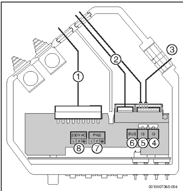
Bild 228 Anschlussbox
