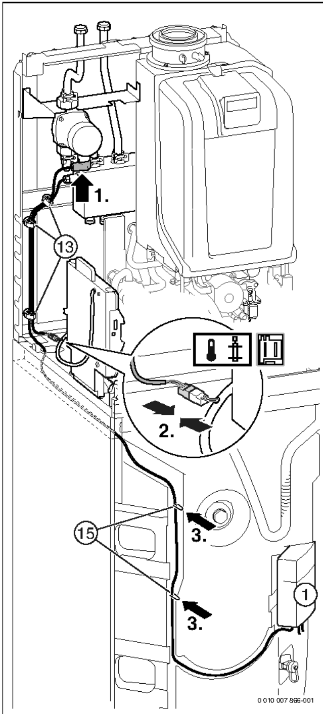
Bild 111 GB.192...iT150...-Geräte: Anschluss Heizungspumpe ungemischter Heizkreis und Hydraulische Weiche
