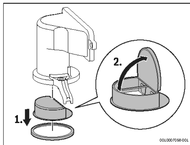
Bild 263 Rückschlagklappe in der Mischeinrichtung
