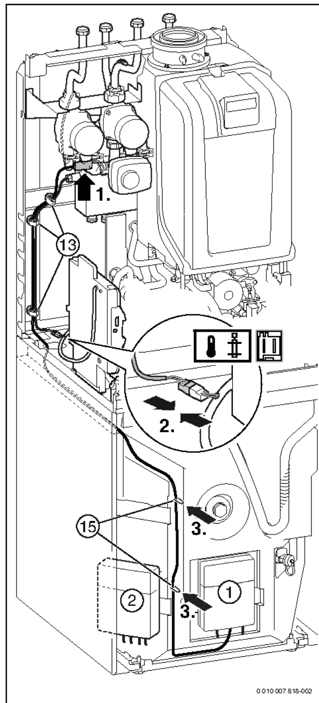
Bild 140 GB.192...iT100...Geräte: Anschluss Heizungspumpe ungemischter Heizkreis und Hydraulische Weiche
