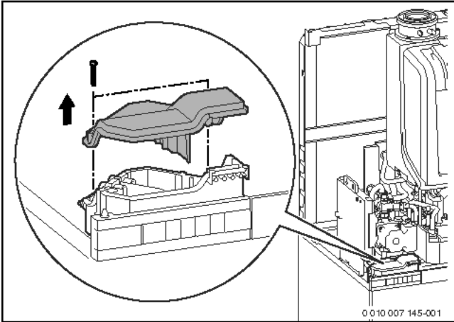
Bild 67 Abdeckung der Anschlussbox entfernen
