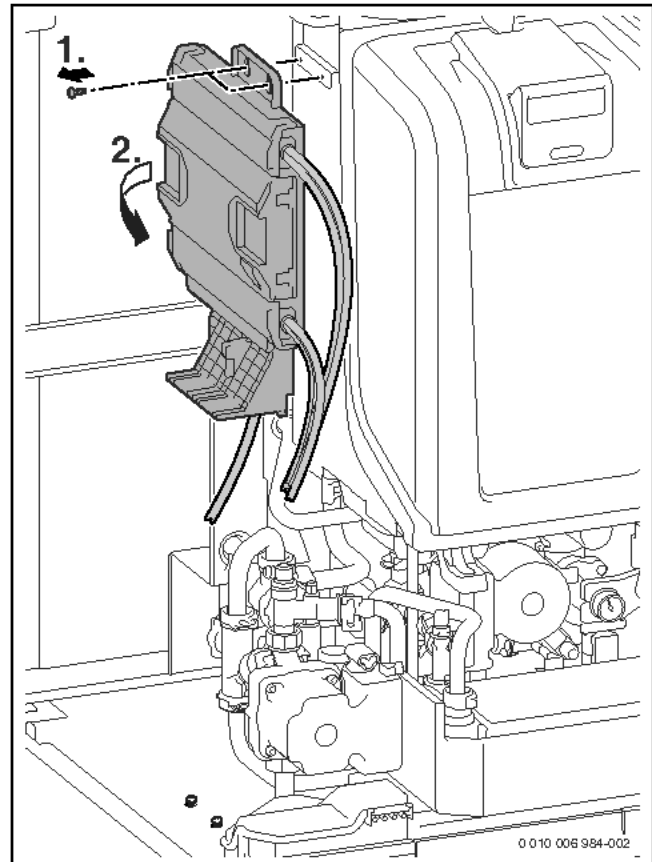
Bild 62 Steuergerät abnehmen
