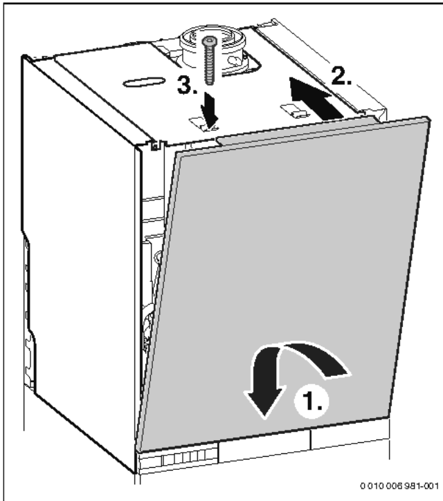
Bild 240 Vordere Verkleidung einhängen und mit Schraube aus Liefer- umfang sichern
