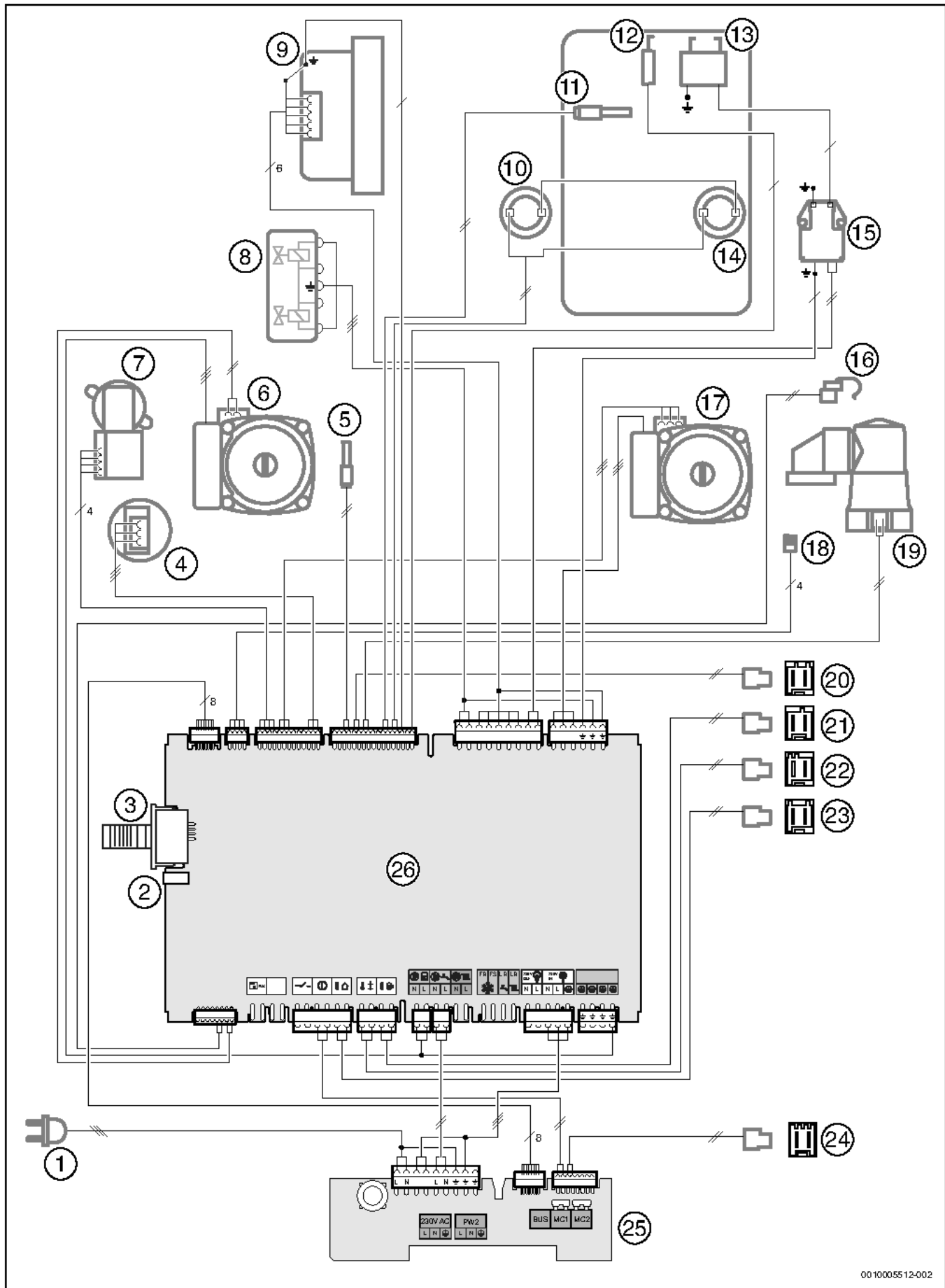
Bild 273 Elektrische Verdrahtung
