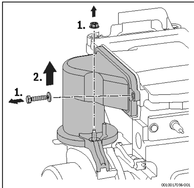
Bild 262 Mischeinrichtung ausbauen
