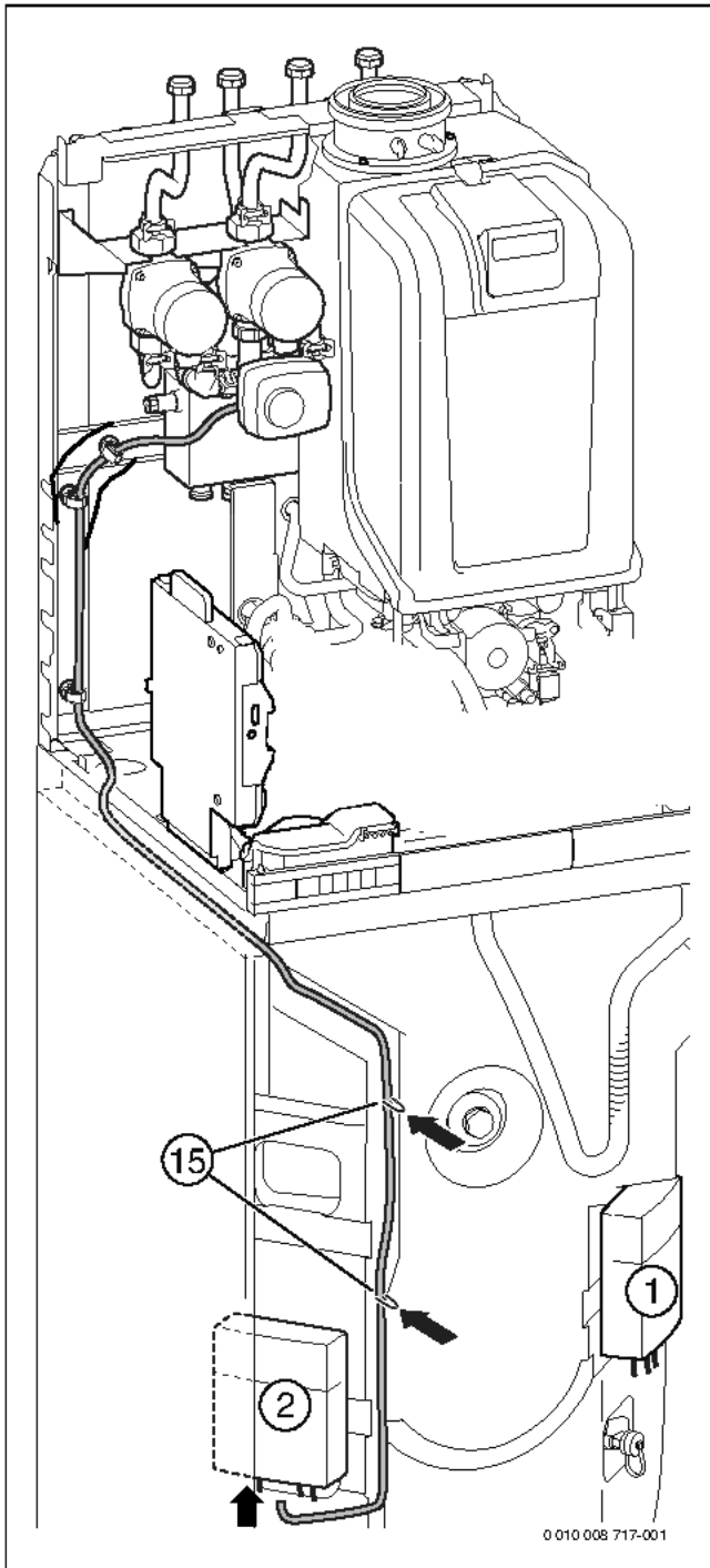
Bild 143 GB.192...iT150...-Geräte: Anschluss Mischermotor
