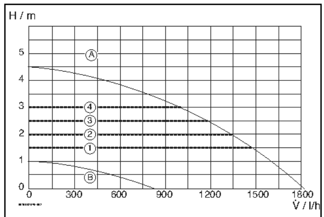
Bild 274 Pumpenkennfelder und Pumpenkennlinien
