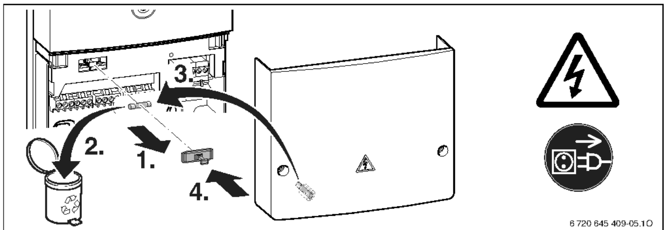
Bild 272 Sicherung vom Modul tauschen
