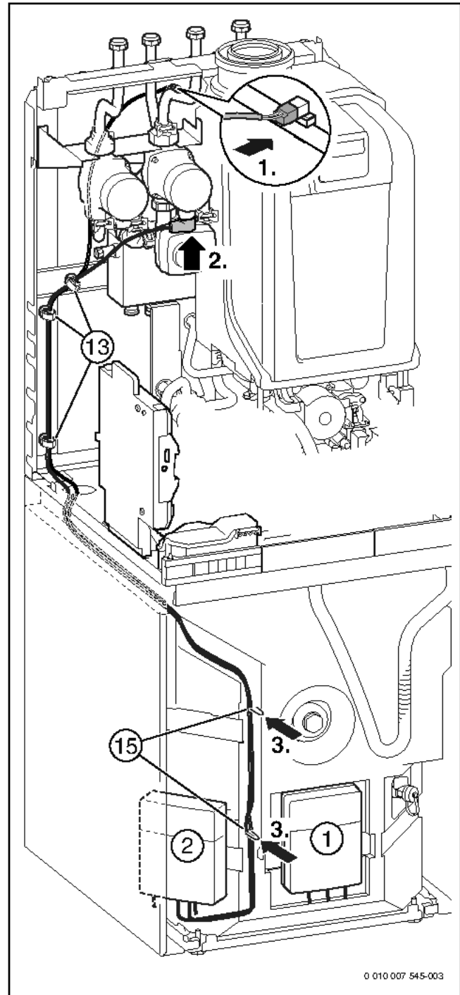
Bild 142 GB.192...iT100...-Geräte: Anschluss Heizungspumpe gemischter Heizkreis und Temperaturfühler
