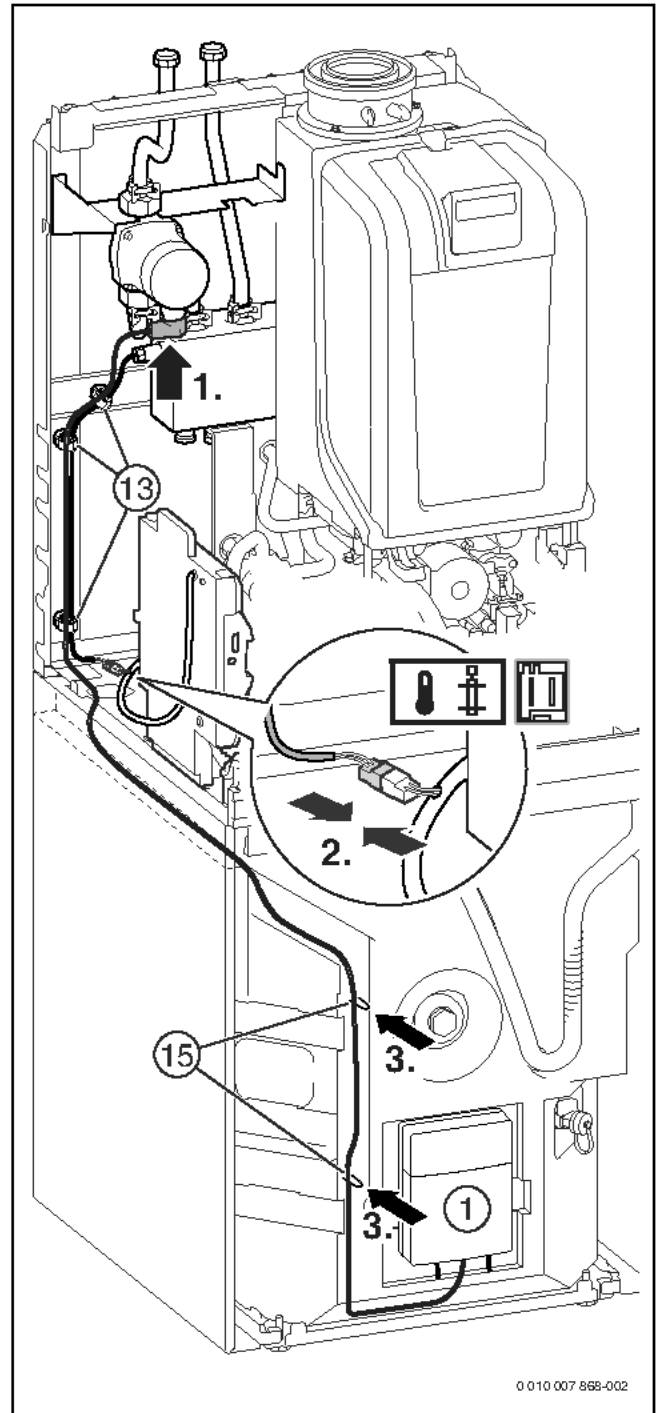
Bild 112 GB.192...iT100...-Geräte: Anschluss Heizungspumpe ungemischter Heizkreis und Hydraulische Weiche
