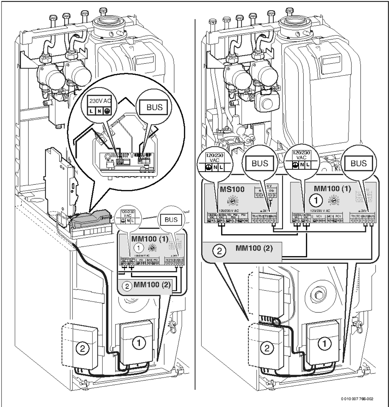
Bild 148 GB.192-...iT100...-Geräte: Anschluss ohne Modul MS100 (links) und mit Modul MS100 (rechts) durchschleifen
