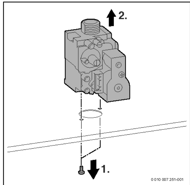
Bild 268 Gasarmatur ausbauen
