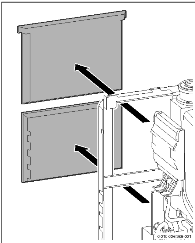
Bild 71 Wärmedämmungen an der Rückseite abnehmen
