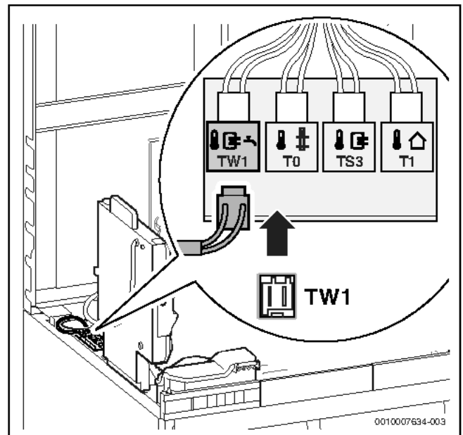
Bild 66 Speichertemperaturfühler anschließen
