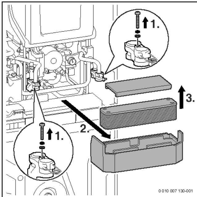
Bild 264 Plattenwärmetauscher ausbauen
