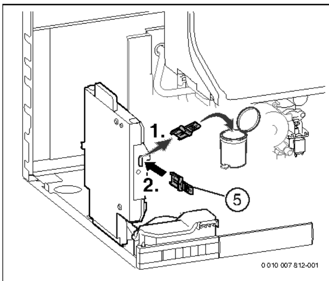
Bild 152 KIM tauschen
