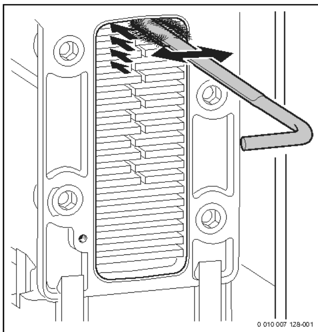
Bild 257 Wärmeblock mit Bürste reinigen
