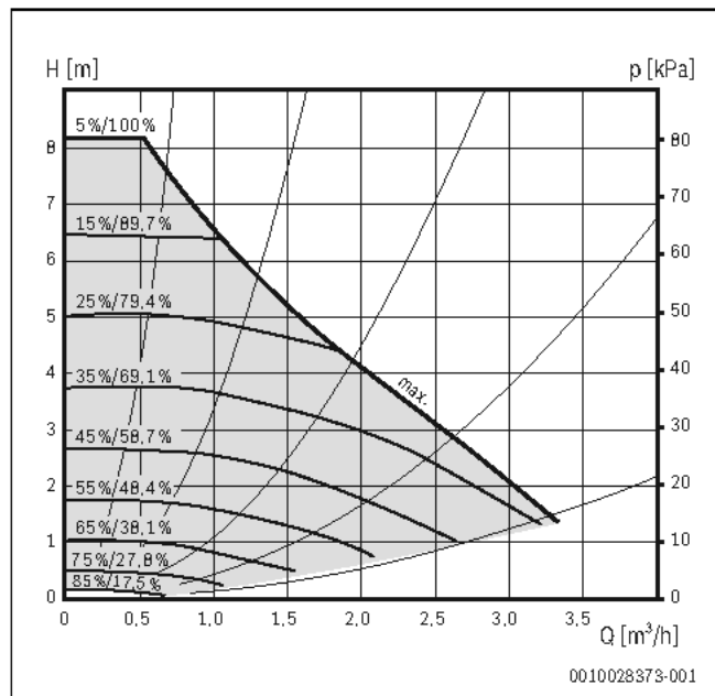
Bild 275 Pumpenkennfelder und Pumpenkennlinien der Solarpumpe Wilo Para ST 15/7-50/iPWM 2, Drehzahlbereich 20–100 %, Volumenstrombereich 0–16,5 l/min
