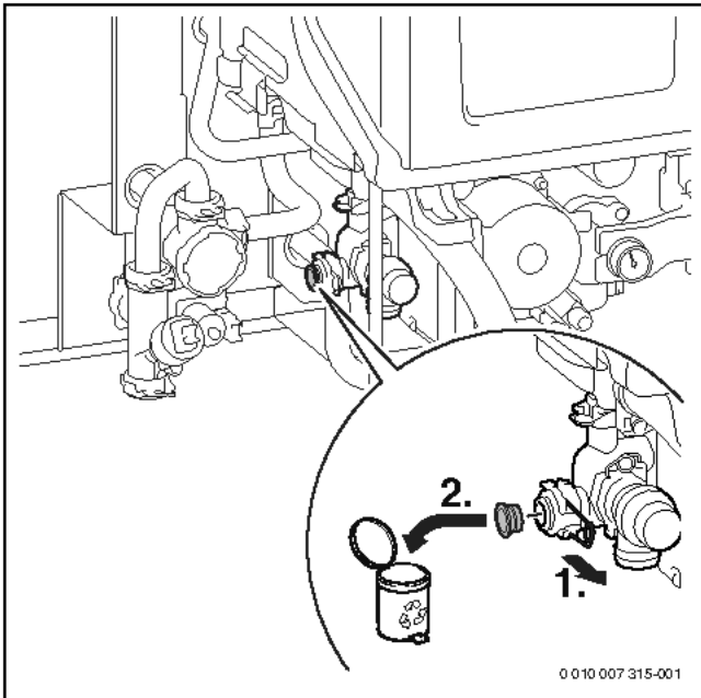
Bild 149 Stopfen entfernen
