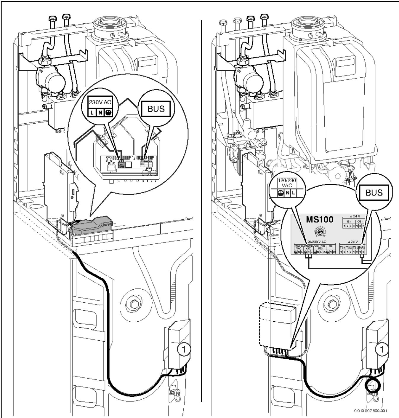
Bild 113 GB.192...IT150...-Geräte: Anschluss ohne Modul MS100 (links) und mit Modul MS100 (rechts)
