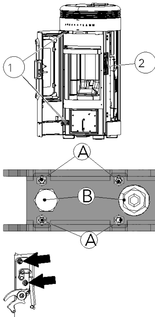
Abb. 37: Feuerraumtür einstellen
