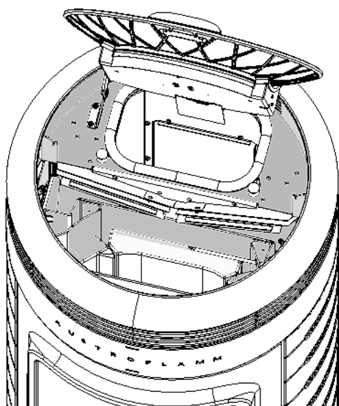
Abb. 47: Hohlraum reinigen
