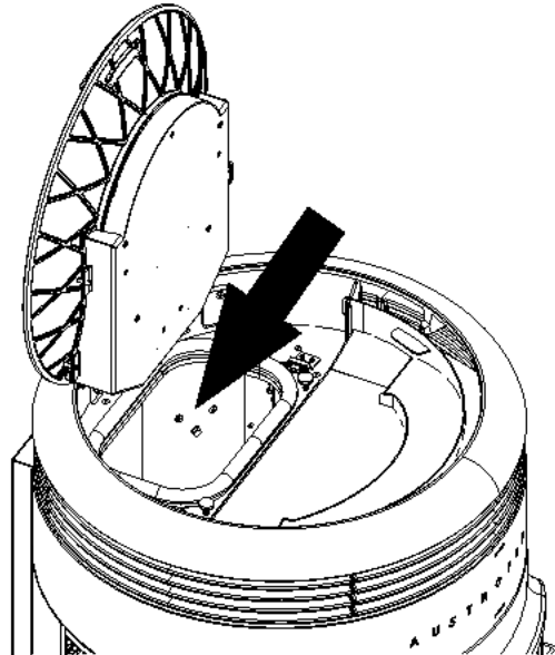
Abb. 23: Pellets füllen
