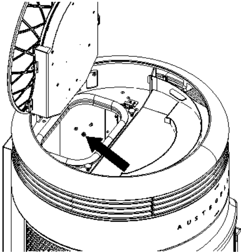
Abb. 39: Schraube lösen
