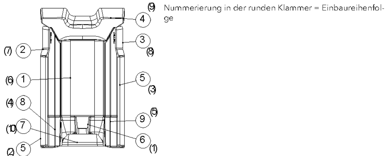
Abb. 14: Keramott einbauen
