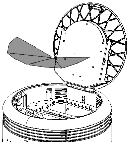
Abb. 44: Strahlungsschutzblech herausnehmen
