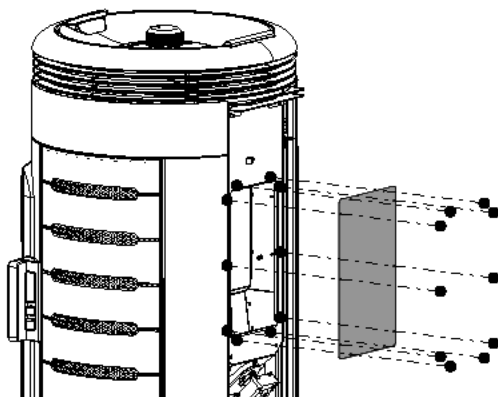
Abb. 16: Abdeckung abmontieren
