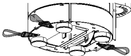
Abb. 6: Transporthilfe
