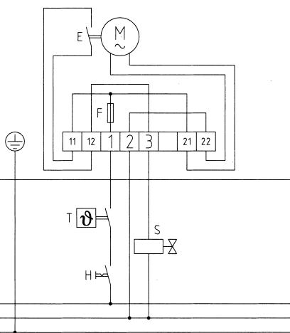
Schematische Darstellung einer Feuerstätte
