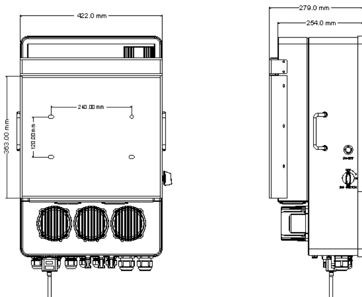
Abmessungen des Wechselrichters
