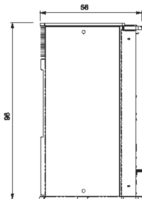
ВИД СБОКУ
