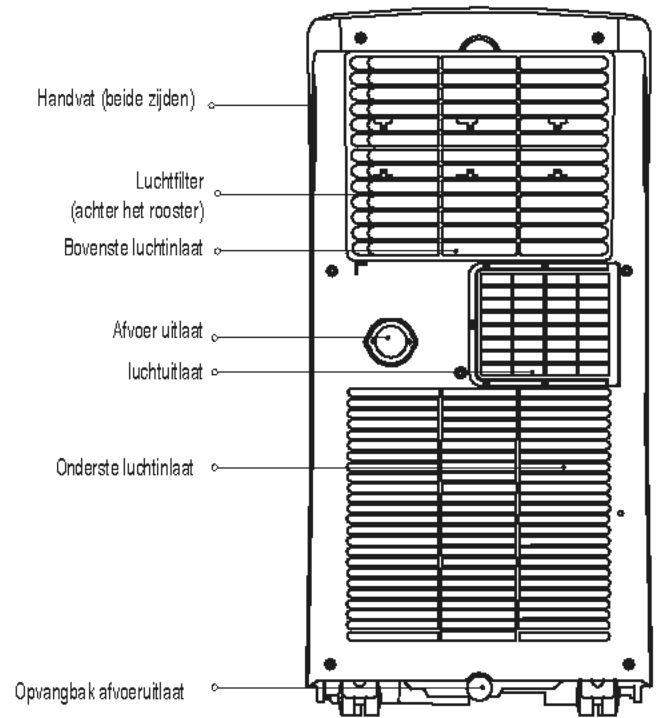
achterkant
