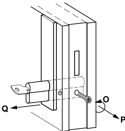
Abb. 4: Austausch des Schließzylinders
