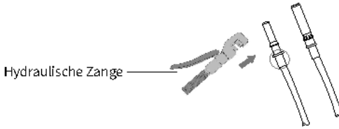
Abb. 3.4 Klemmen Sie den Kontaktstift an den Draht
