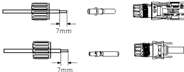
Abb. 3.3 Demontieren Sie die Überwurfmutter des Steckers
