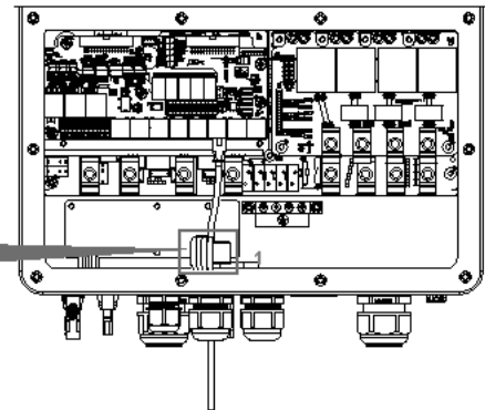
Abb. 3.6 DC-Eingangsanschluss
