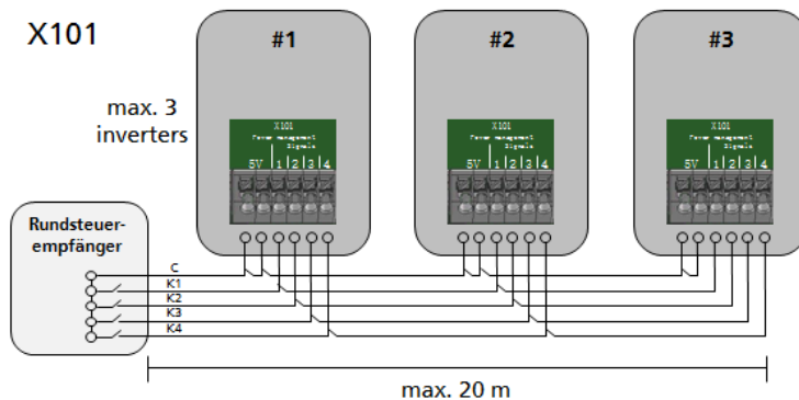
Abb. 6-5 Anschluss Rundsteuerempfänger
