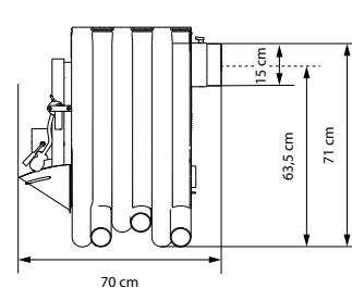
Bruno Pyro II mit Herdplatte / with hob / avec cuisinière / con piano cottura
