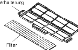
Filterhalterung
