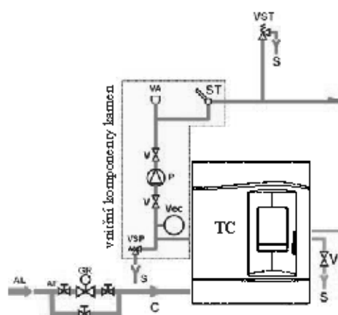
SCHÉMA TOPNÉHO SYSTÉMU S KAMNY A BOJLEREM
