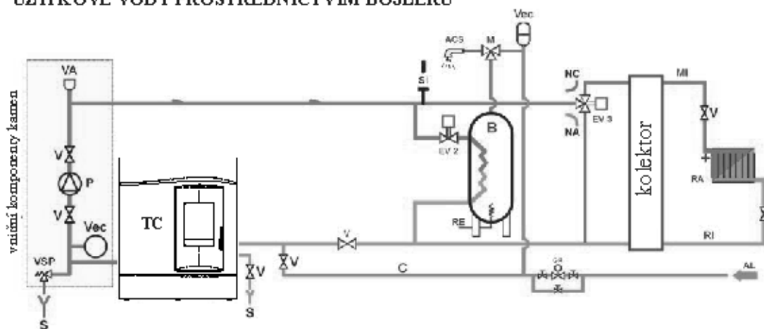
SCHÉMA TOPNÉHO SYSTÉMU S KAMNY JAKOŽTO JEDINÝM ZDROJEM TEPLA S VÝROBOU TEPLÉ UŽITKOVÉ VODY PROSTŘEDNICTVÍM BOJLERU
