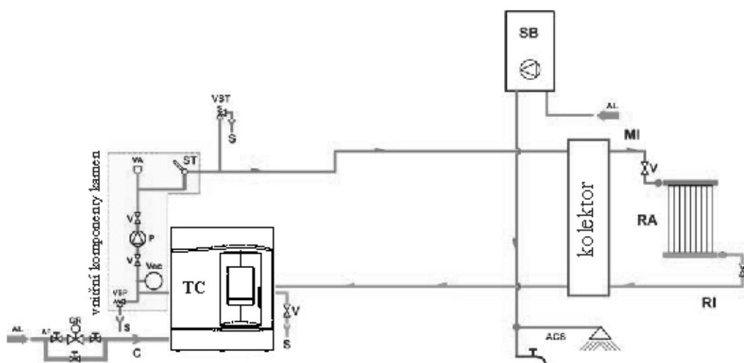
SCHÉMA TOPNÉHO SYSTÉMU S KAMNY JAKOŽTO JEDINÝM ZDROJEM TEPLA S VÝROBOU TEPLÉ UŽITKOVÉ VODY PROSTŘEDNICTVÍM BOJLERU
