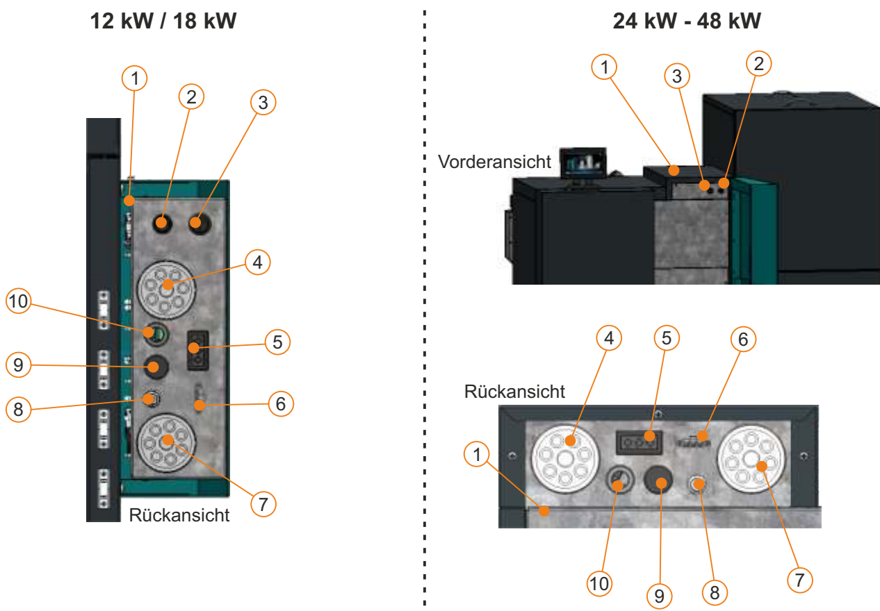
Bild 4. Kesselregelung (Schalter, Stromanschlüsse, Kabelführung)
