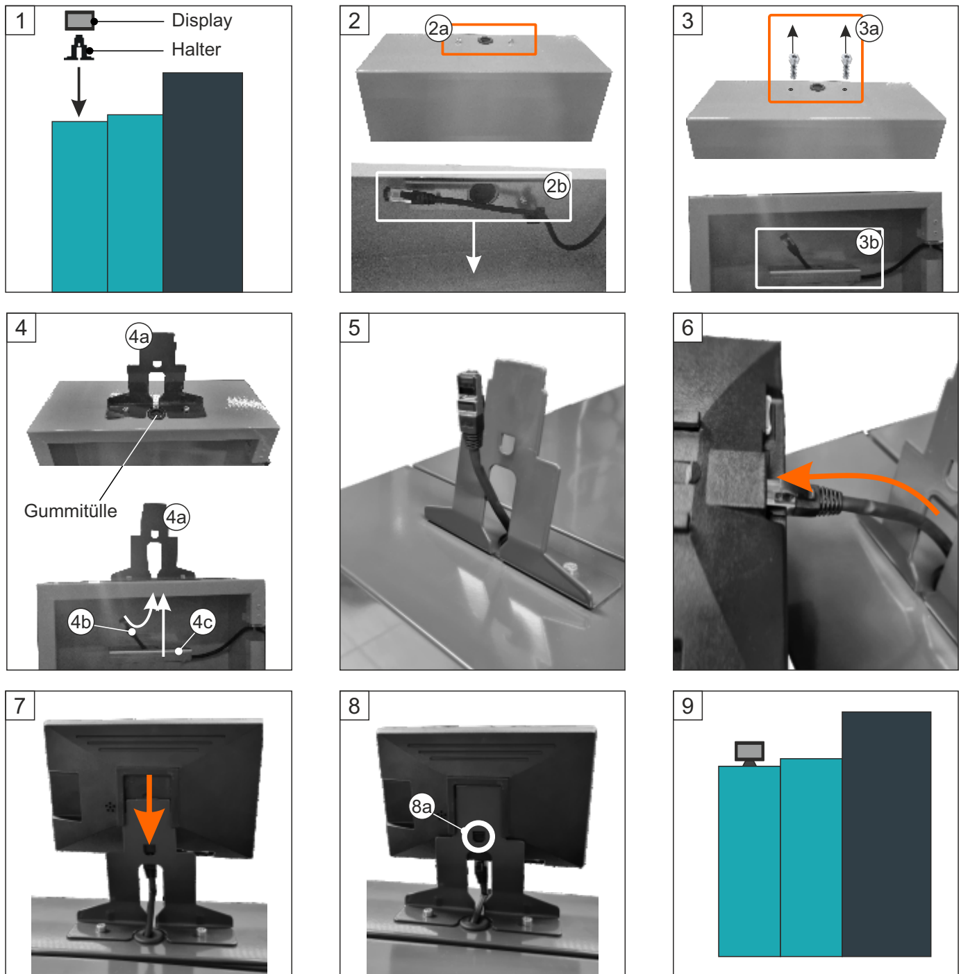
Bild 8. Montage des Halters und des 7"-Displays der Kesselsteuerung (18-48 kW)
