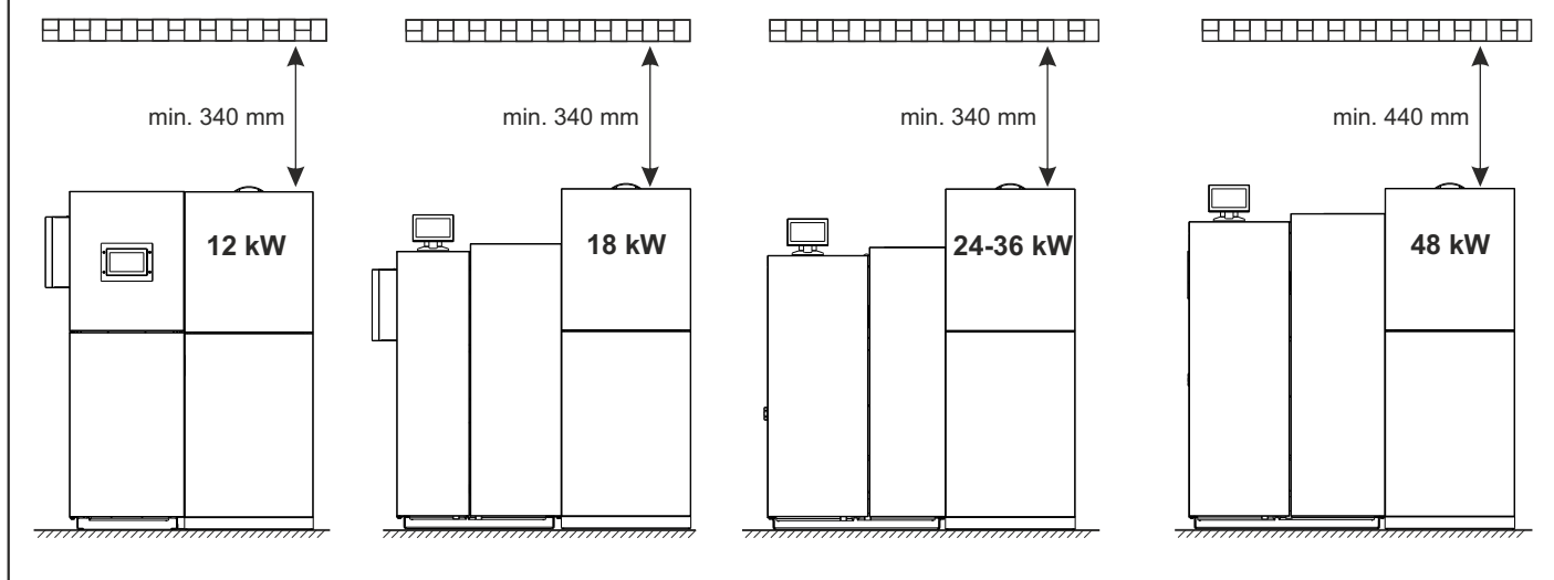
Bild 2b. Erforderlicher Mindestabstand des Heizkessels zur Heizraumdecke.
