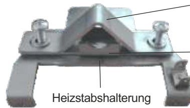
Heizstabshalterung mit Klemme Durchmesser Ø 20 mm
