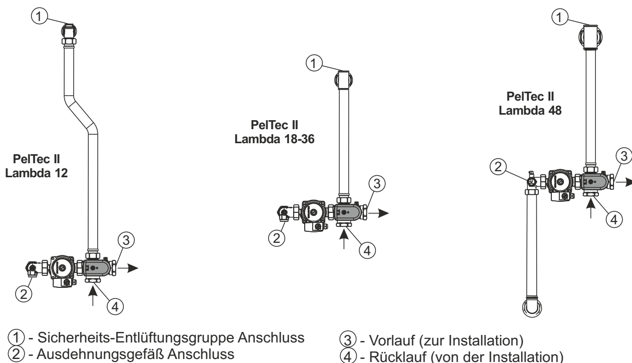
Bild 3. Anschlüsse des Kessels zum Anschluss an das geschlossene Heizungssystem
