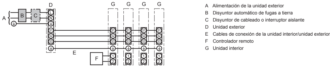
Sistema doble/triple/cuádruple simultáneo
