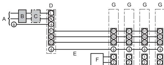
Praca równoczesna w układzie twin/triple/quadruple
