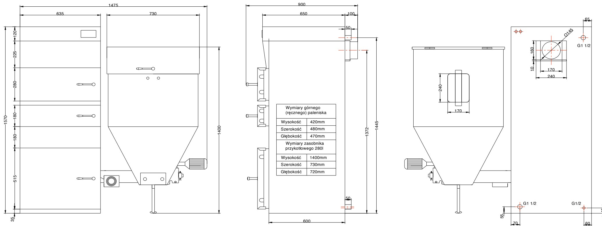
bb. Nr. 4. Abmessungen des Kessels LING DUO 50kW mit einem Vorratsbehälter 280 L.
