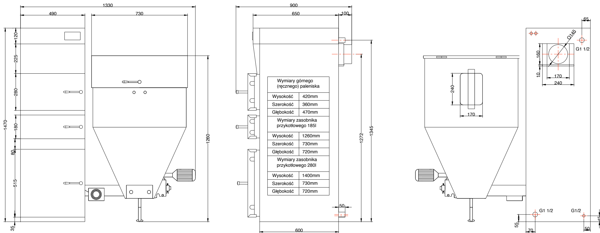
Abb. Nr. 2. Abmessungen des Kessels LING DUO 25kW mit einem Vorratsbehälter 185 L (erhältlich mit 280 L).
