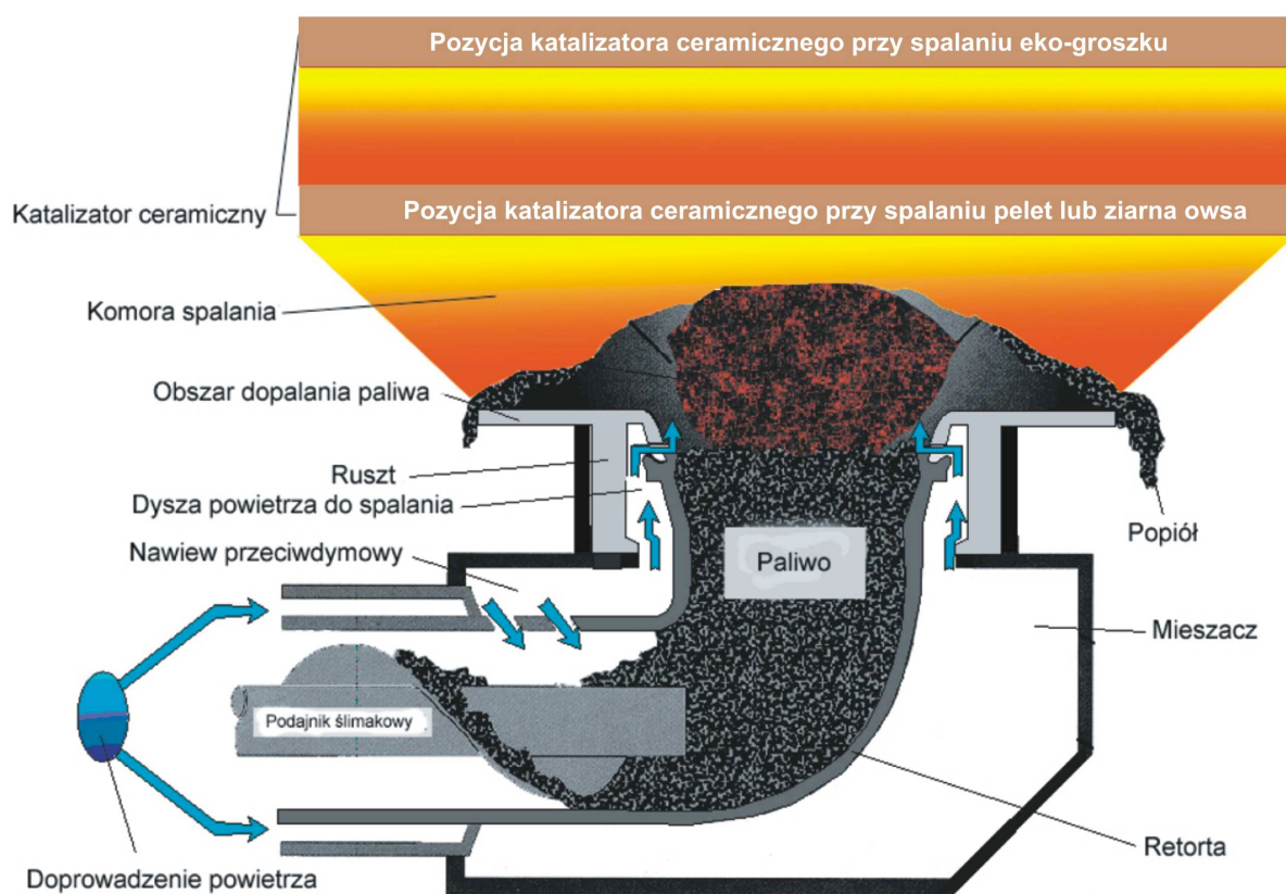
Abb. Nr. 7. Übersichtsschema des Retortenbrennraums bei der Kohlenverbrennung und die Einbauweise der Katalysatoren.
