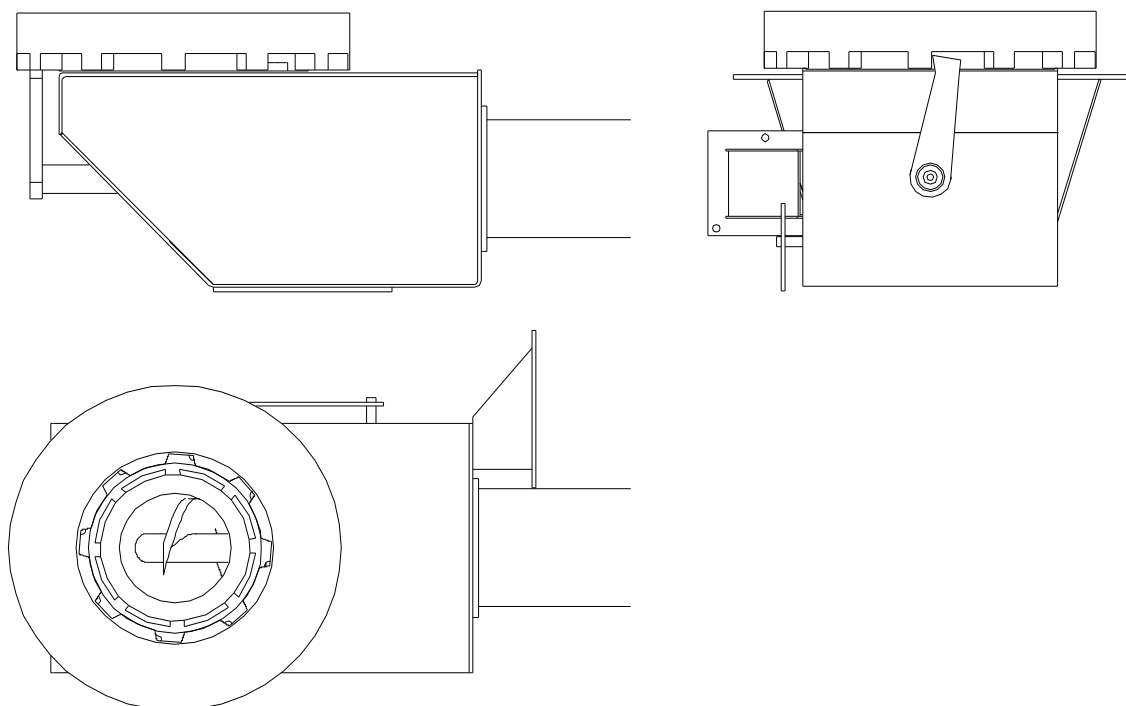
Abb. Nr. 8. Übersichtsschema des Retortenbrennraums mit Drehtrost (auf Wunsch Ling Duo 15 - 35 ).
