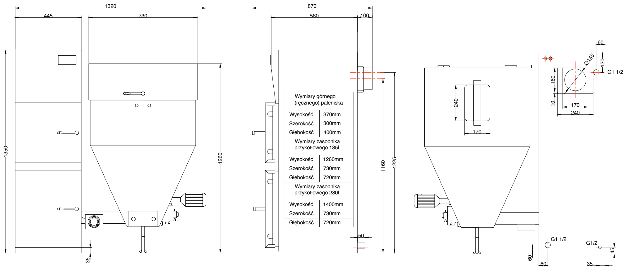
Abb. Nr. 1. Abmessungen des Kessels LING DUO 15kW mit einem Vorratsbehälter 185 L.
