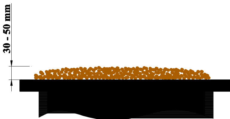
Abbildung 14. Lage der Nusskohle auf dem Retortenbrenner beim Kesselbetrieb.
