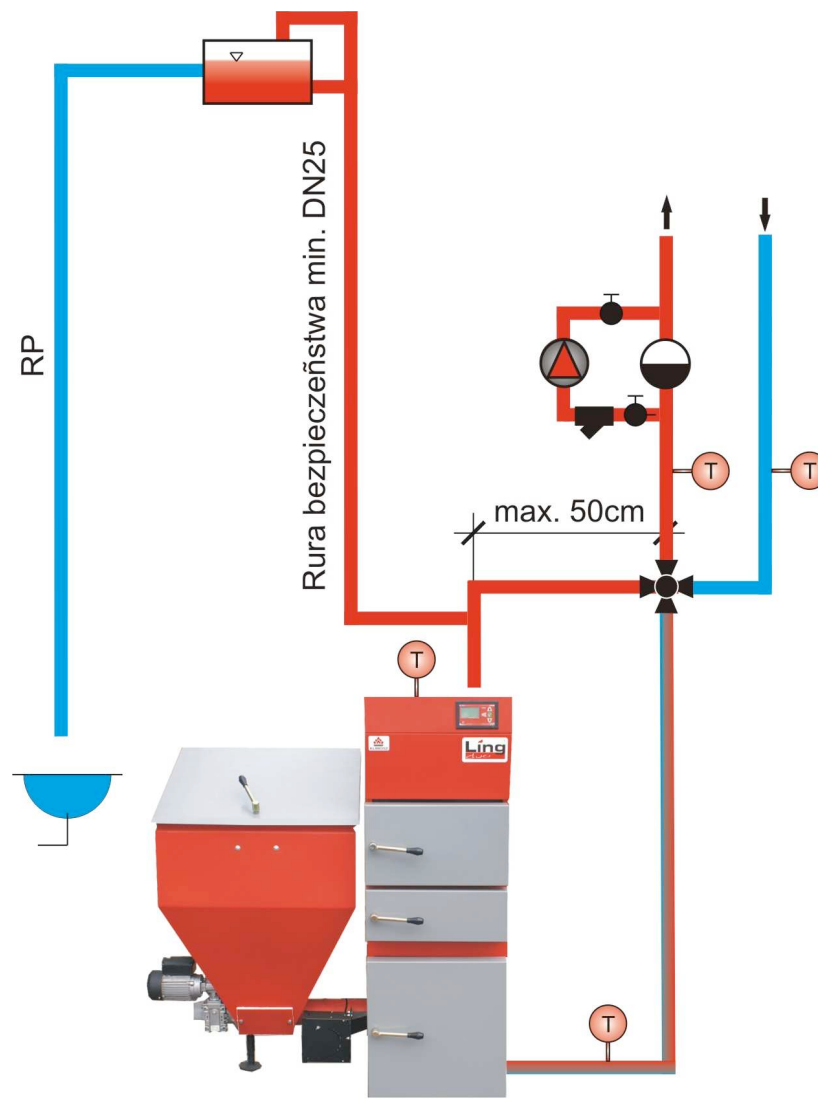
Abb. Nr. 13. Montage 4-Wege-Ventil – Richtlinien
