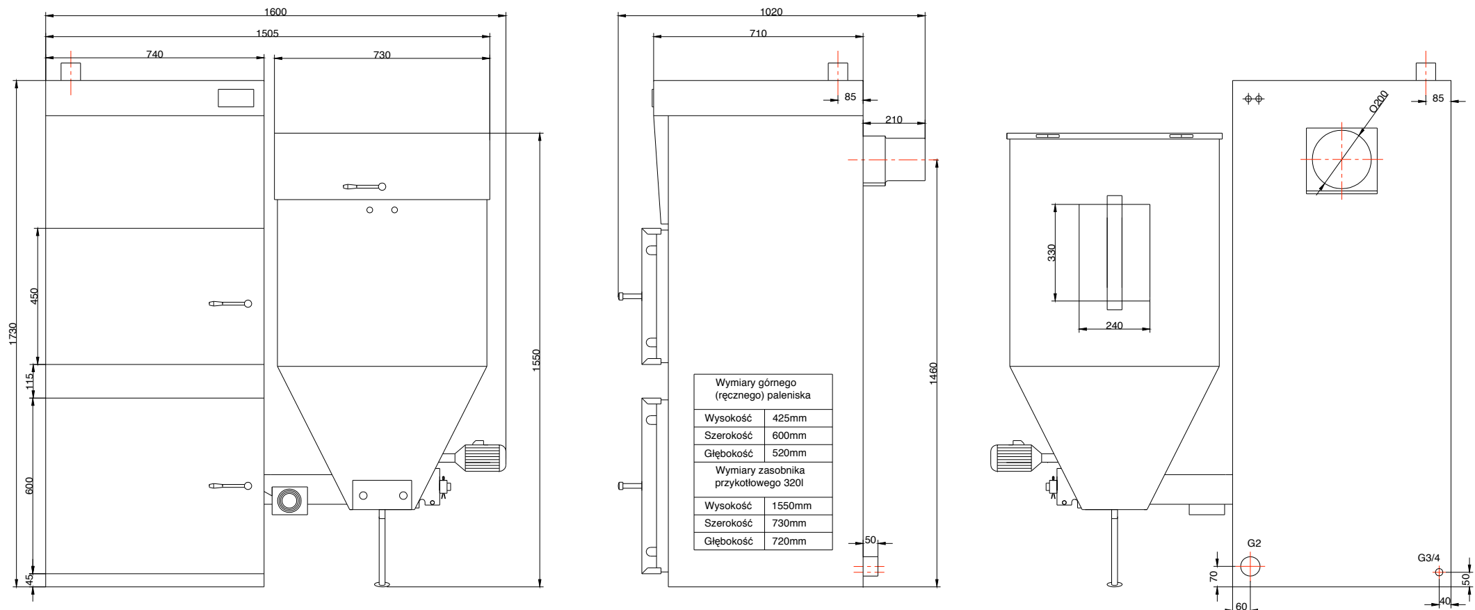
Abb. Nr. 5. Abmessungen des Kessels LING DUO 75kW mit einem Vorratsbehälter 320 L (erhältlich mit 920 L).
