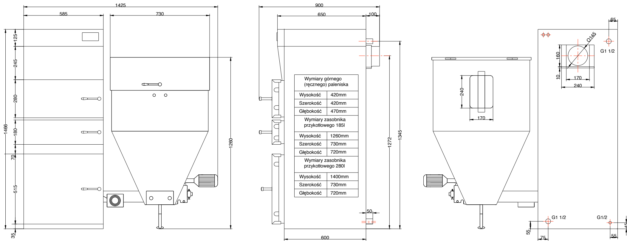
Abb. Nr. 3. Abmessungen des Kessels LING DUO 35kW mit einem Vorratsbehälter 185 L (erhältlich mit 280 L).
