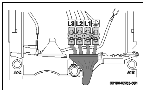
Fig. 105 Raccordement intérieur pour câble court
