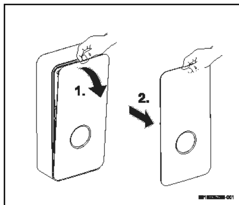
Bild 9 Frontblende abnehmen
