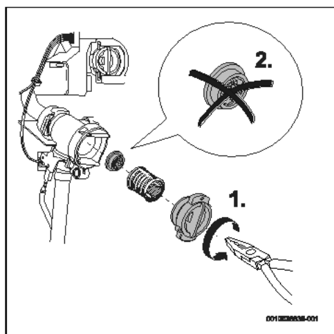
Bild 54 Durchflussbegrenzer entfernen.
