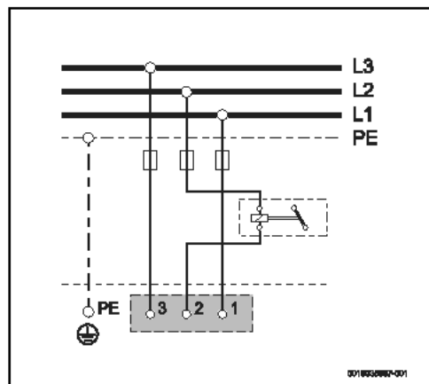
Bild 39 Schaltplan
