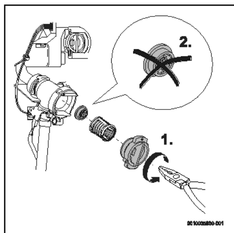
Fig. 110 retirer le limiteur de débit.
