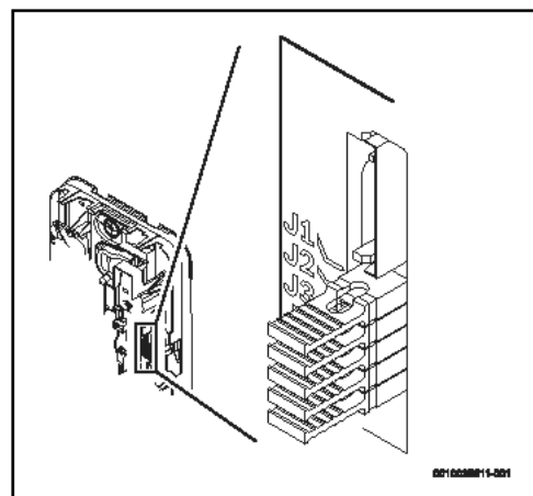
Fig. 93 Cavaliers électroniques fournis
