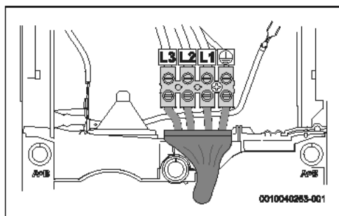
Bild 49 Anschluss unten kurze Kabel
