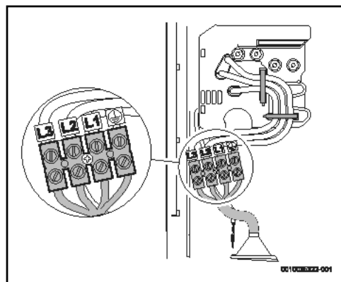
Bild 41 Anschluss unten
