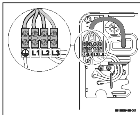
Bild 40 Anschluss oben
