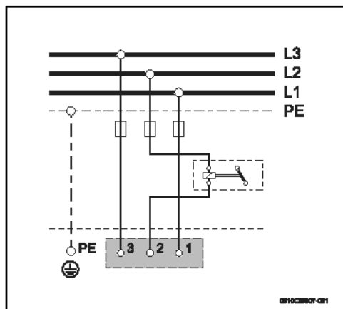
Fig. 95 Schéma de câblage
