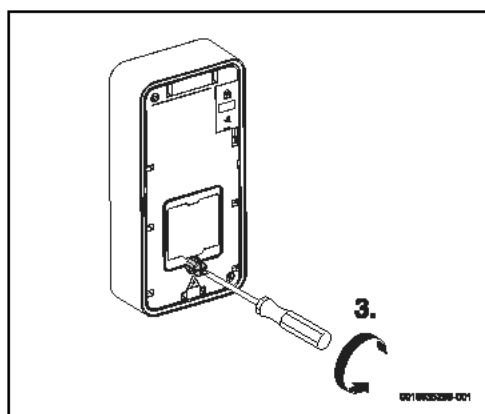
Bild 12 Schraube lösen
