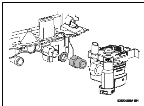
Fig. 87 Bague supplémentaire
