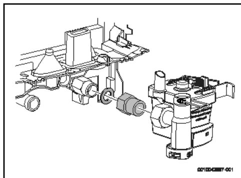
Bild 30 Zusätzliche Buchse
