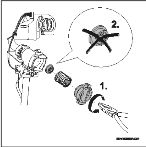
Bild 58 Durchflussbegrenzer entfernen.
