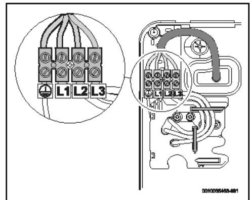
Bild 44 Anschluss oben
