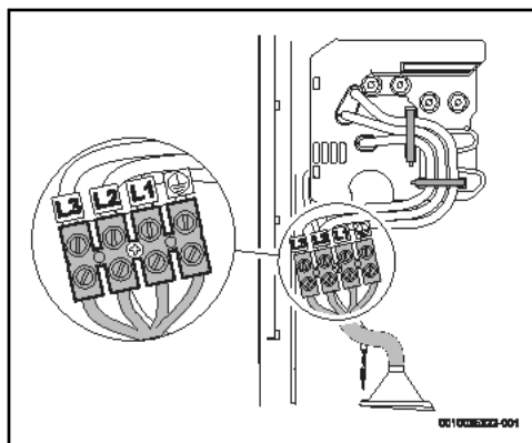
Fig. 96 Raccord inférieur
