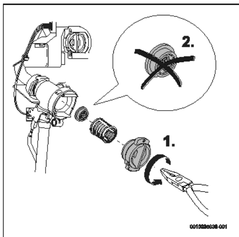
Fig. 109 retirer le limiteur de débit.
