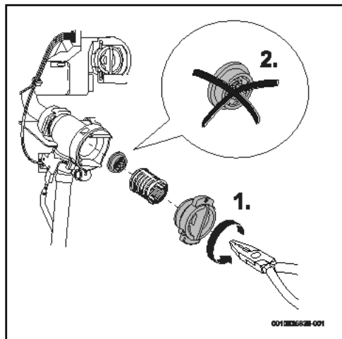
Rys. 163 Usunięcie ogranicznika przepływu.
