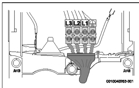
Fig. 104 Raccordement inférieur pour câble court
