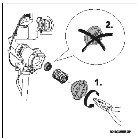
Bild 55 Durchflussbegrenzer entfernen.
