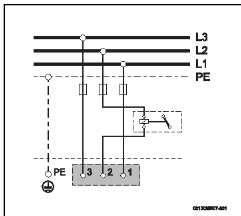
Fig. 94 Schéma de câblage
