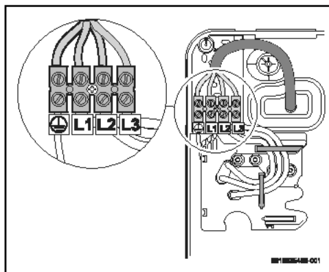
Fig. 95 Raccord supérieur
