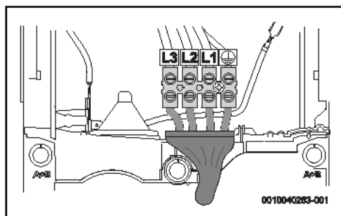
Rys. 151 Przyłącze od dołu na krótkie kable
