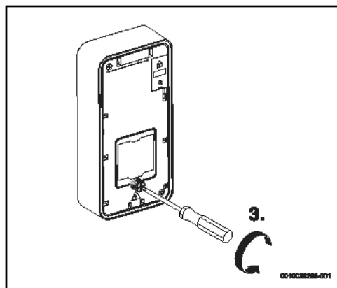
Rys. 119 Wykręcanie śruby
