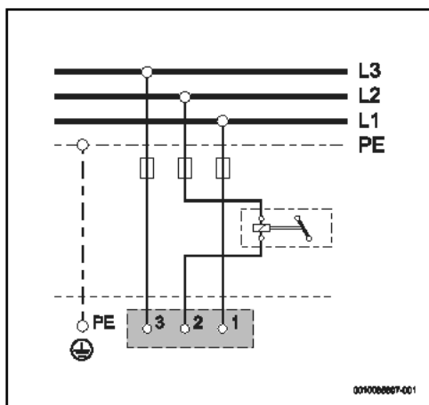
Rys. 148 Schemat elektryczny
