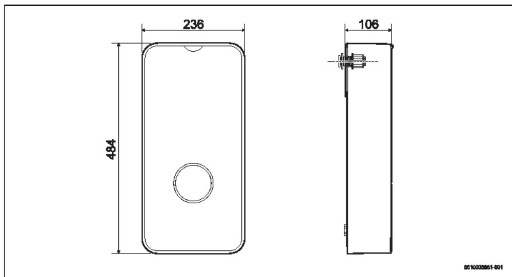
Rys. 100 Wymiary wmm
