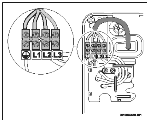
Fig. 85 Raccord supérieur
