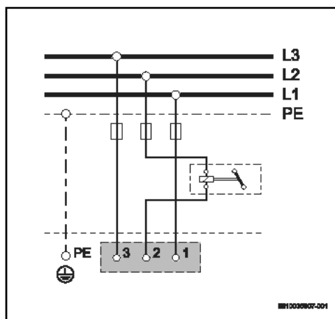
Fig. 84 Schéma de connexion
