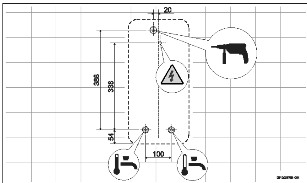
Rys. 101 Wymiary wmm
