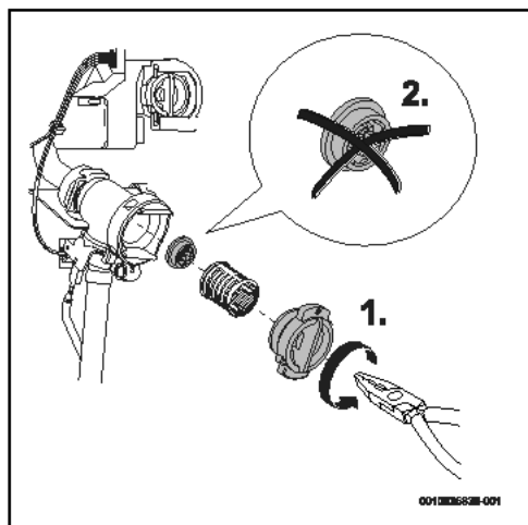
Rys. 148 Usunięcie ogranicznika przepływu.
