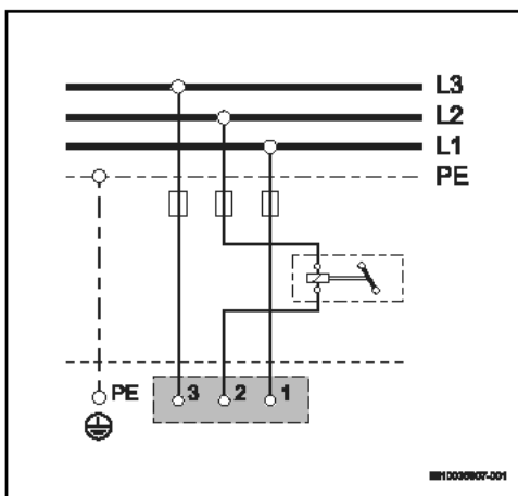
Bild 35 Schaltplan
