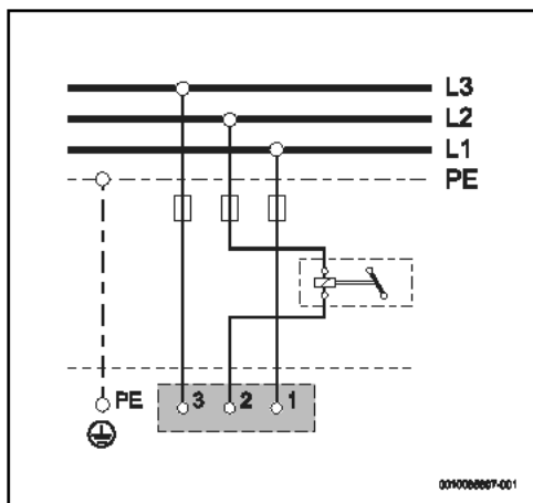
Rys. 133 Schemat połączeń
