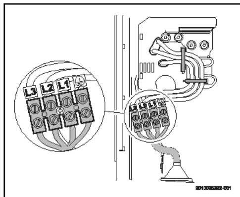
Fig. 86 Raccord inférieur
