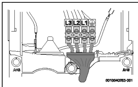
Fig. 94 Raccordement intérieur pour câble court
