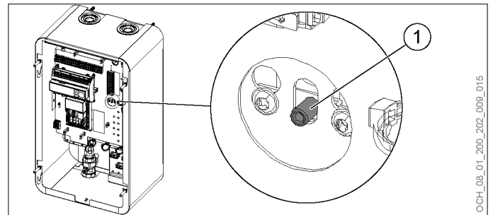
1 Reset-Taster des Sicherheitstemperaturbegrenzers
