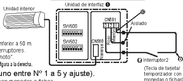
Conexión de tecla de tarjeta temporizador con monedas o fichas
