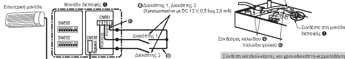
Σύνδεση κλειδιού-κάρτας και χρονοδιακόπτη-κερματοδέκτη
