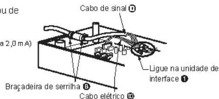
Ligação da chave de cartão ou temporizador de moeda
