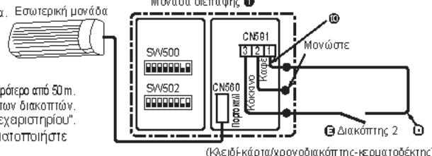
Σύνδεση κλειδιού-κάρτας και χρονοδιακόπτη-κερματοδέκτη
