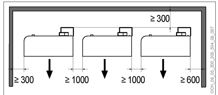
► Installation mehrerer Außenteile zwischen zwei Wänden.
