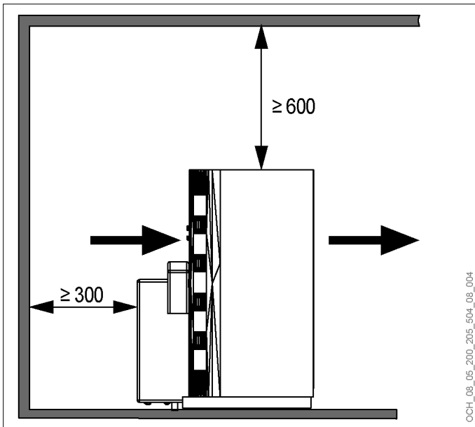
► Installation zwischen zwei Wänden.
