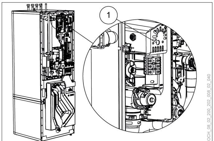
1 Reset-Taster des Sicherheitstemperaturbegrenzers
