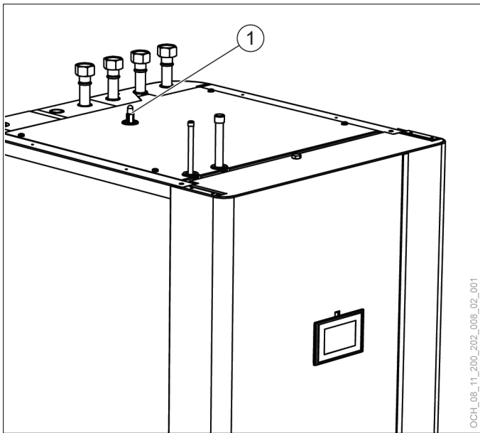
1 Verbrauchsanzeige der Magnesiumanode
