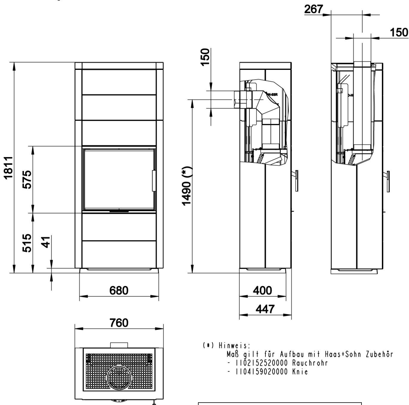
Abbildung 30: Abmessungen
