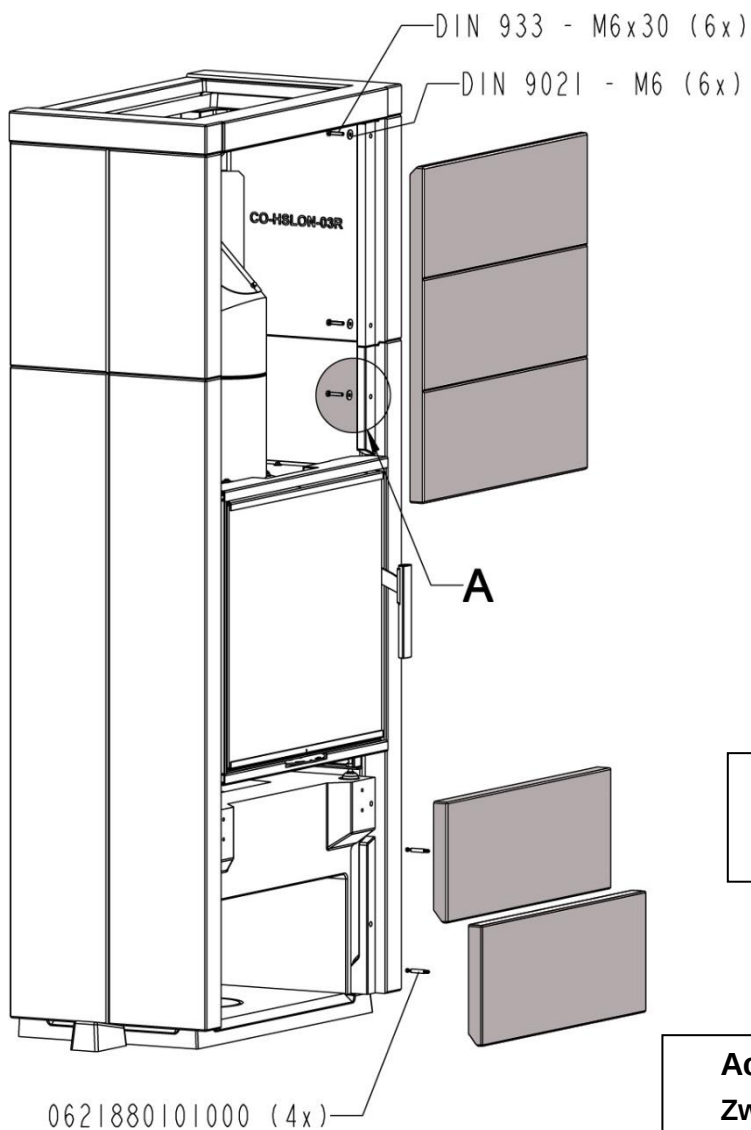
Abbildung 13-14: Montage der Fronplatten oben und unten
