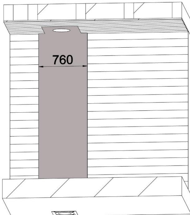
Abbildung 27: Rauchrohranschluss- Brandschutzvorgaben
