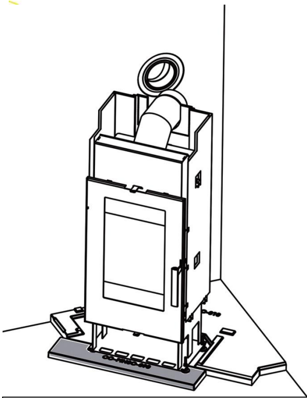
Abbildung 6: Montageplatte auflegen, Einsatz vorrücken
